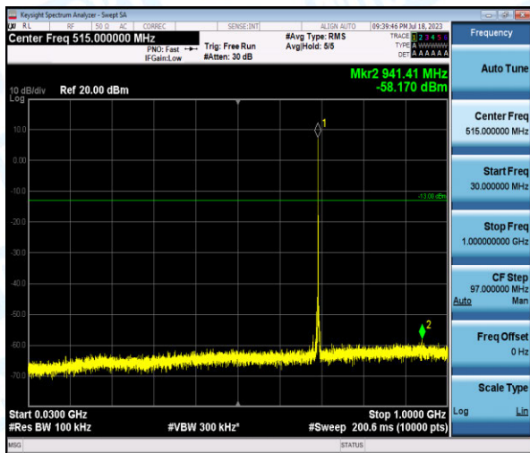
Band12-10MHz-QPSK-23060-1-0-Low-30-1000--58.17-PASS
