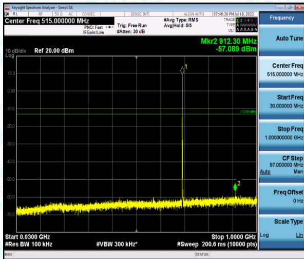
Band12-1.4MHz-QPSK-23017-1-0-Low-30-1000--57.09-PASS
