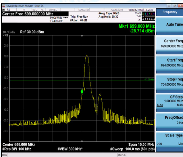
Band12-5MHz-QPSK-23035-1-0-Low--25.71-PASS
