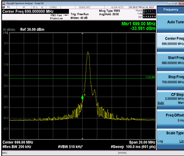
Band12-10MHz-QPSK-23060-1-0-Low--33.59-PASS
