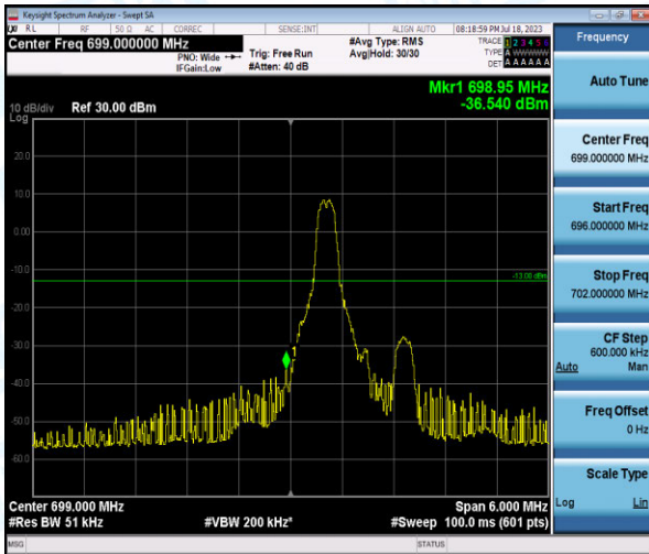
Band12-3MHz-QPSK-23025-1-0-Low--36.54-PASS
