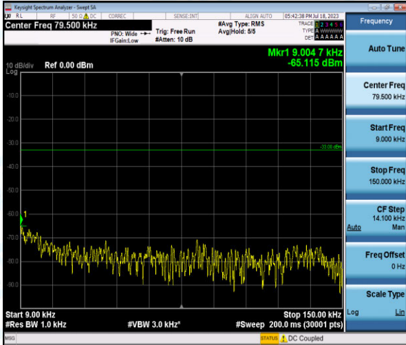
Band5-5MHz-QPSK-20425-1-0-Low-0.009-0.15--65.12-PASS
