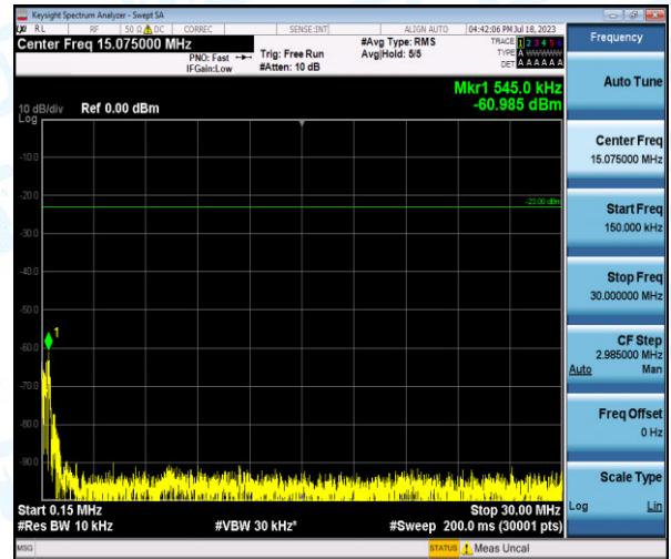
Band5-3MHz-QPSK-20415-1-0-Low-0.15-30--60.99-PASS
