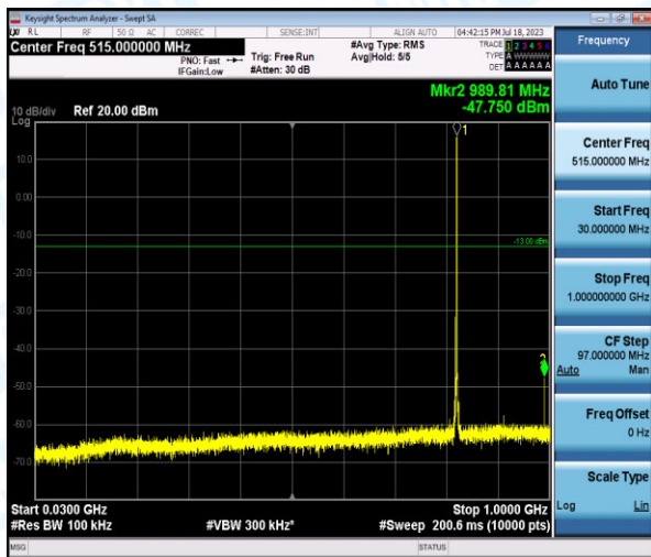
Band5-3MHz-QPSK-20415-1-0-Low-30-1000--47.75-PASS
