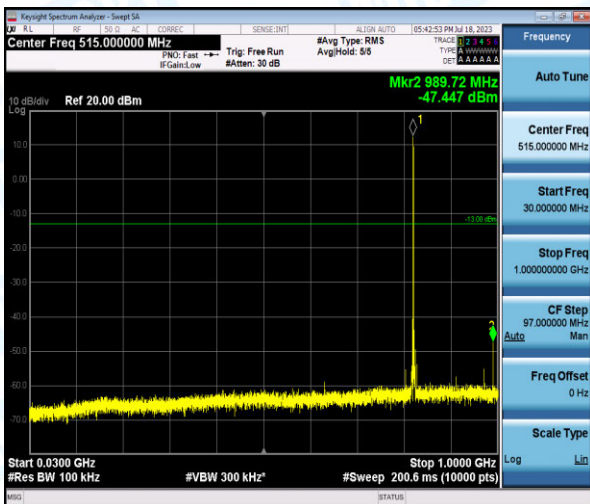
Band5-5MHz-QPSK-20425-1-0-Low-30-1000--47.45-PASS
