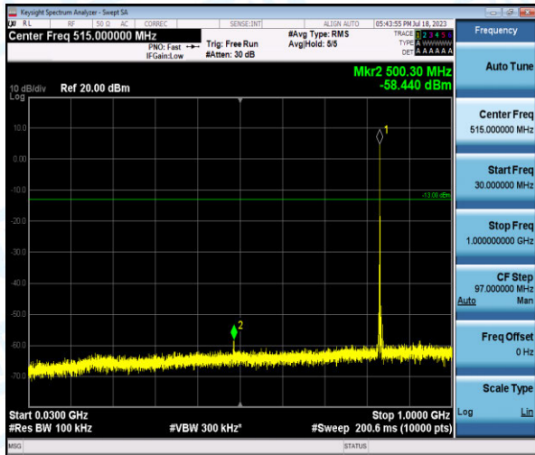
Band5-5MHz-QPSK-20525-1-0-Low-30-1000--58.44-PASS
