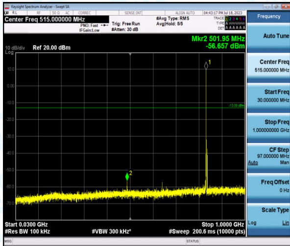
Band5-3MHz-QPSK-20525-1-0-Low-30-1000--56.66-PASS
