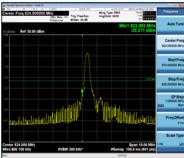
Band5-5MHz-QPSK-20425-1-0-Low--25.27-PASS
