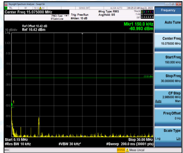
Band4-20MHz-QPSK-20050-1-0-Low-0.15-30--60.99-PASS
