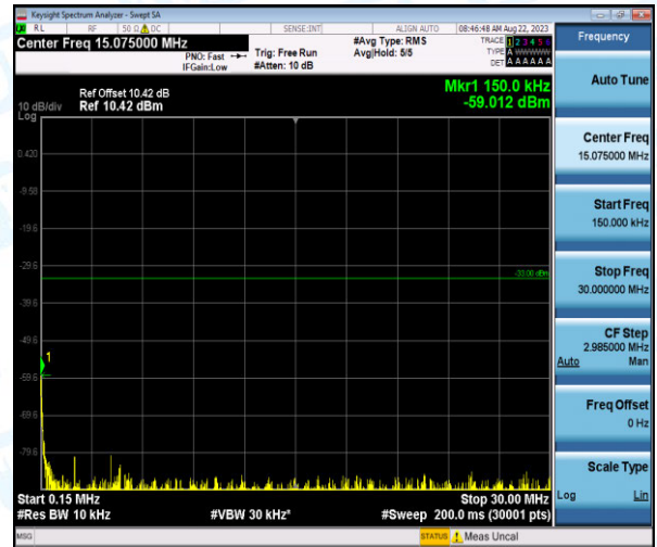
Band4-10MHz-16QAM-20000-1-0-Low-0.15-30--59.01-PASS
