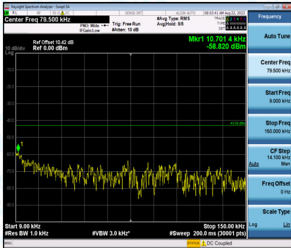
Band4-3MHz-QPSK-19965-1-0-Low-0.009-0.15--58.82-PASS
