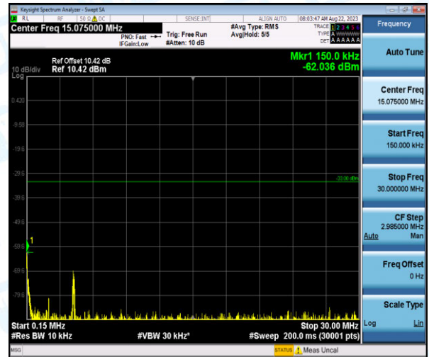
Band4-3MHz-QPSK-19965-1-0-Low-0.15-30--62.04-PASS
