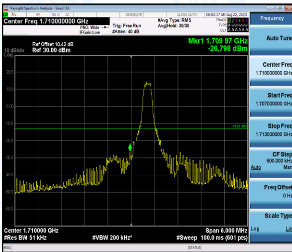
Band4-3MHz-QPSK-19965-1-0-Low--26.80-PASS
