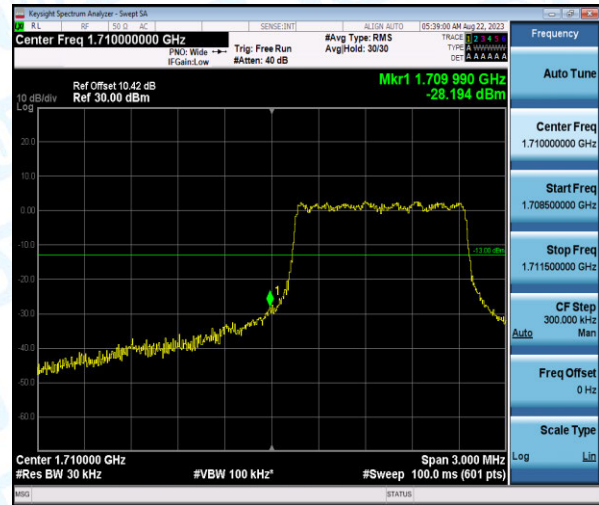
Band4-1.4MHz-QPSK-19957-6-0-Low--28.19-PASS
