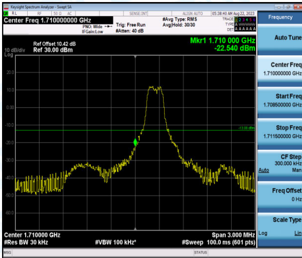
Band4-1.4MHz-QPSK-19957-1-0-Low--22.54-PASS
