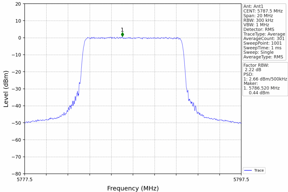
10M_MCH_5787.5MHz_MIMO_NTNV
