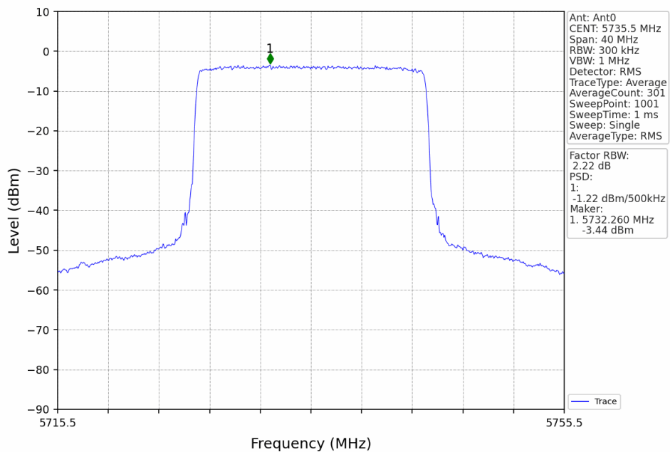
20M_LCH_5735.5MHz_Ant0_NTNV
