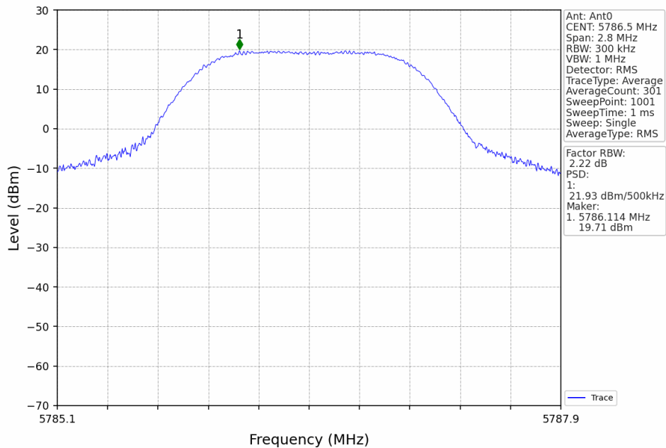
1.4M_MCH_5786.5MHz_Ant0_NTNV
