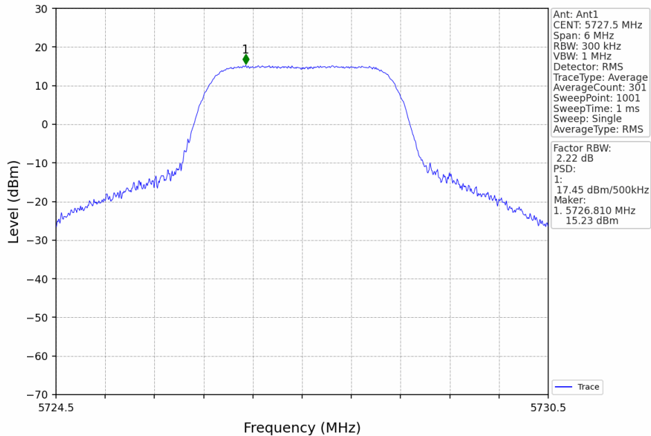
3M_LCH_5727.5MHz_MIMO_NTNV
