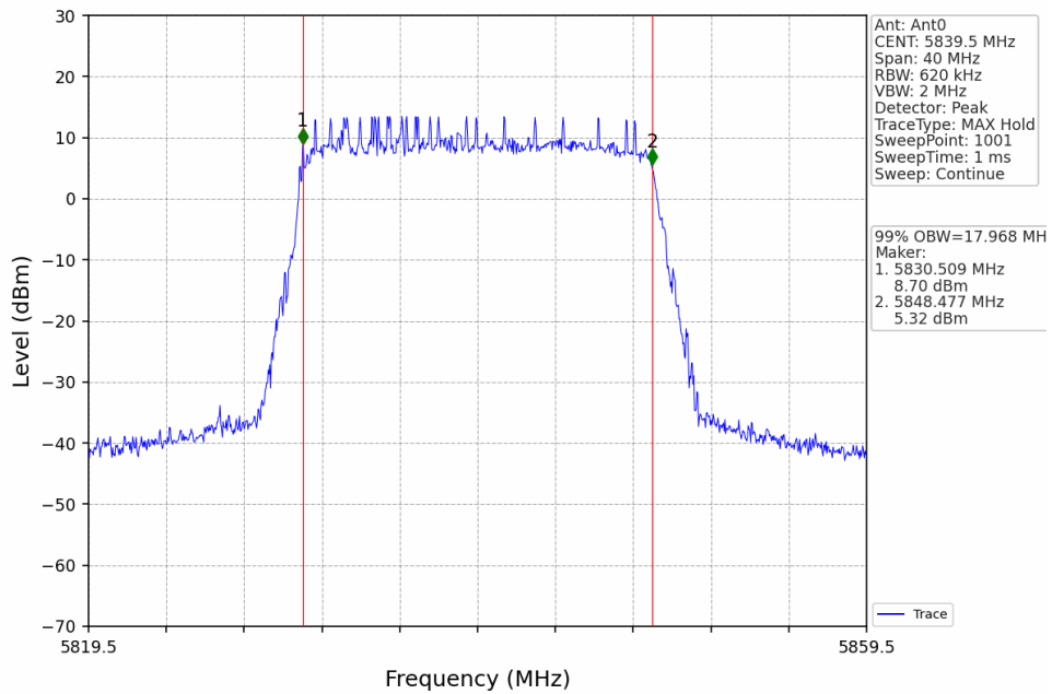
20M_HCH_5839.5MHz_Ant0_NTNV
