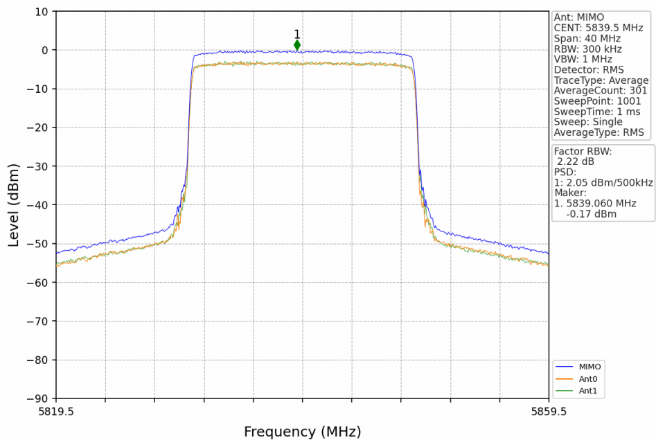
20M_HCH_5839.5MHz_MIMO_NTNV
