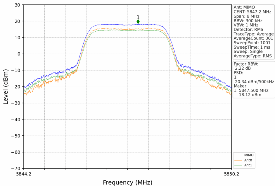
3M_HCH_5847.2MHz_MIMO_NTNV
