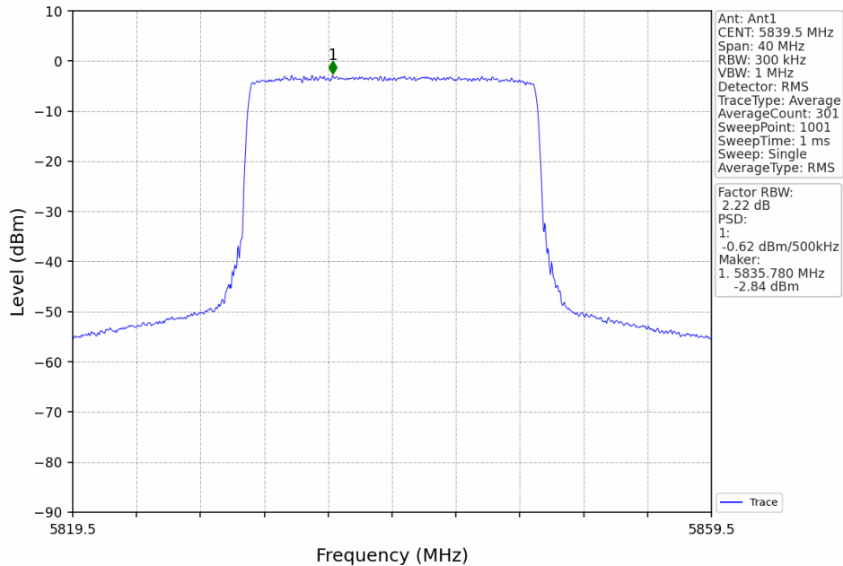
20M_HCH_5839.5MHz_MIMO_NTNV
