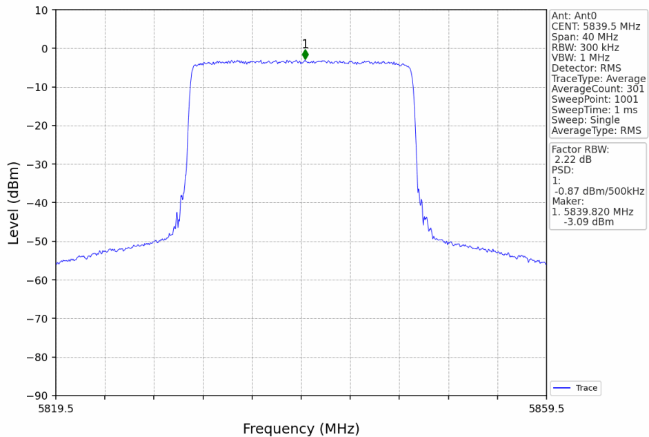
20M_HCH_5839.5MHz_Ant0_NTNV
