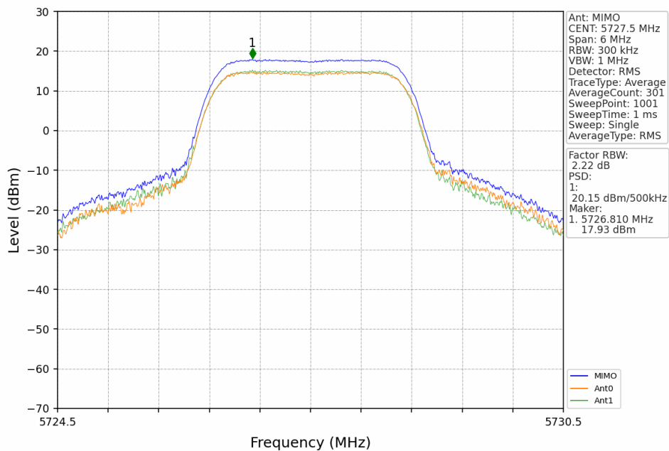
3M_LCH_5727.5MHz_MIMO_NTNV
