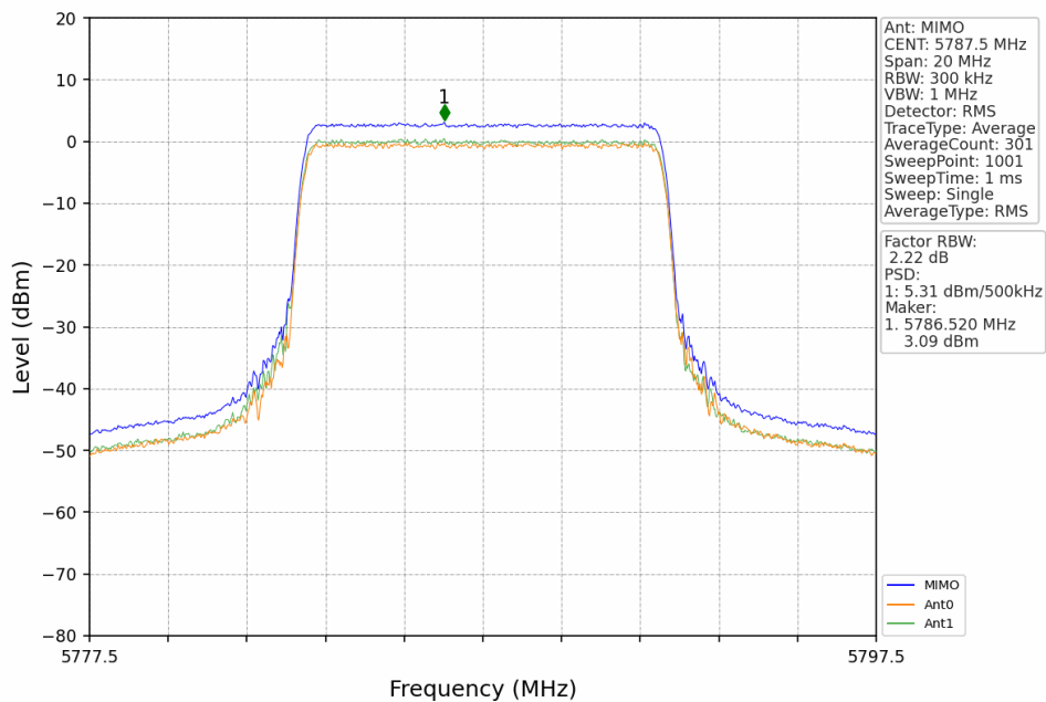
10M_MCH_5787.5MHz_MIMO_NTNV
