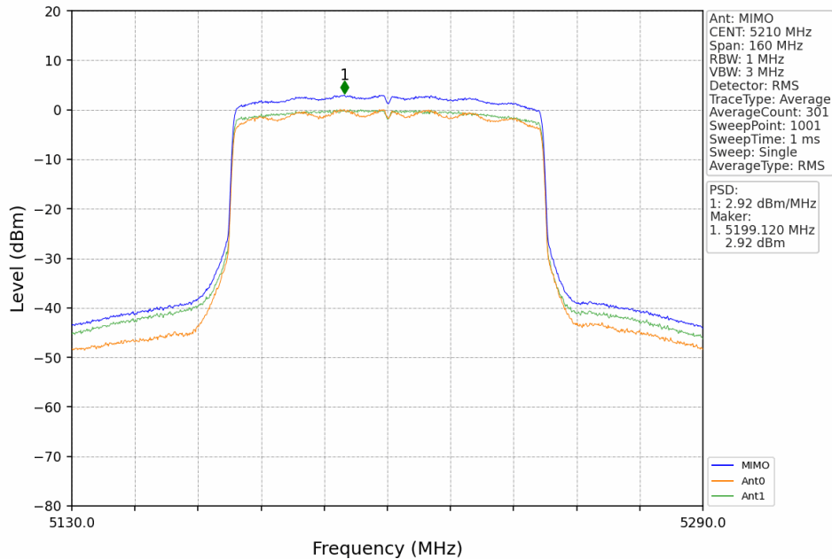
802.11ax(HEW80)_MCH_5210MHz_RU996_Left_MIMO_NTNV
