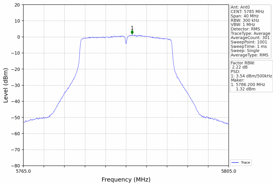
802.11n(HT20)_MCH_5785MHz_Ant0_NTNV
