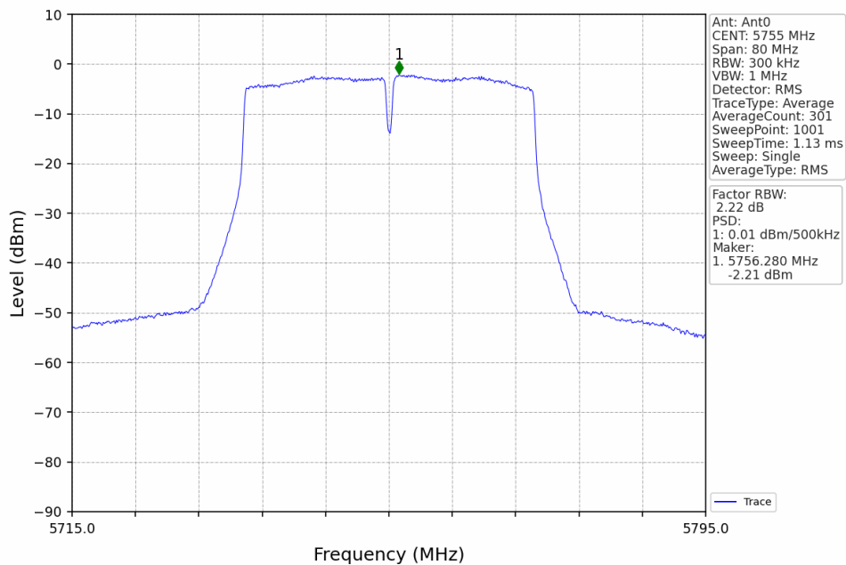
802.11n(HT40)_LCH_5755MHz_Ant0_NTNV
