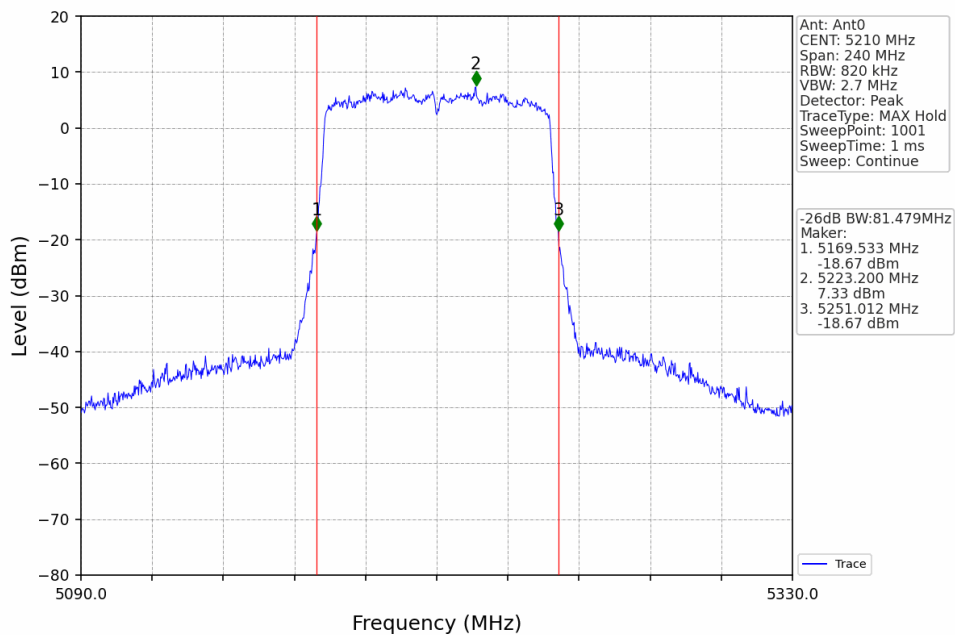
802.11ac(VHT80)_MCH_5210MHz_Ant0_NTNV
