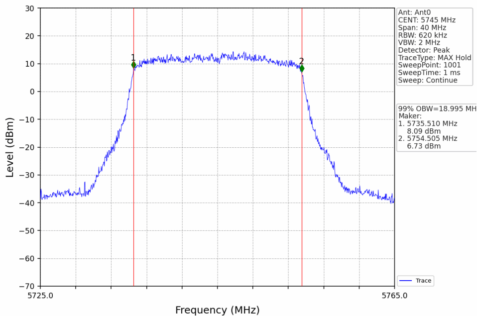
802.11ax(HEW20)_LCH_5745MHz_RU242_Left_Ant0_NTNV
