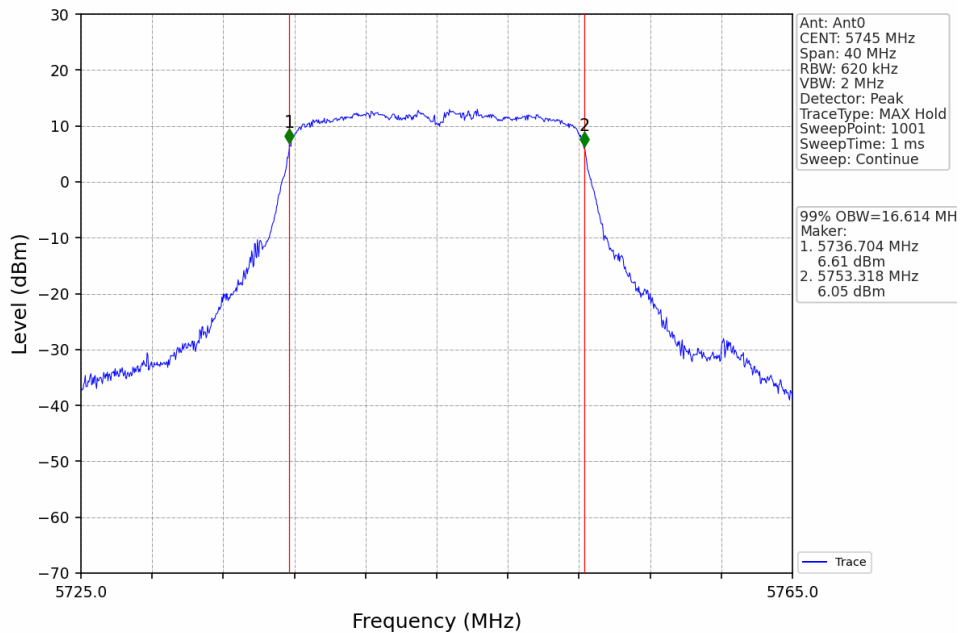
802.11a_LCH_5745MHz_Ant0_NTNV
