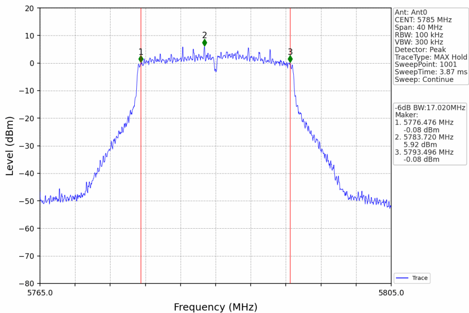
802.11ac(VHT20)_MCH_5785MHz_Ant0_NTNV
