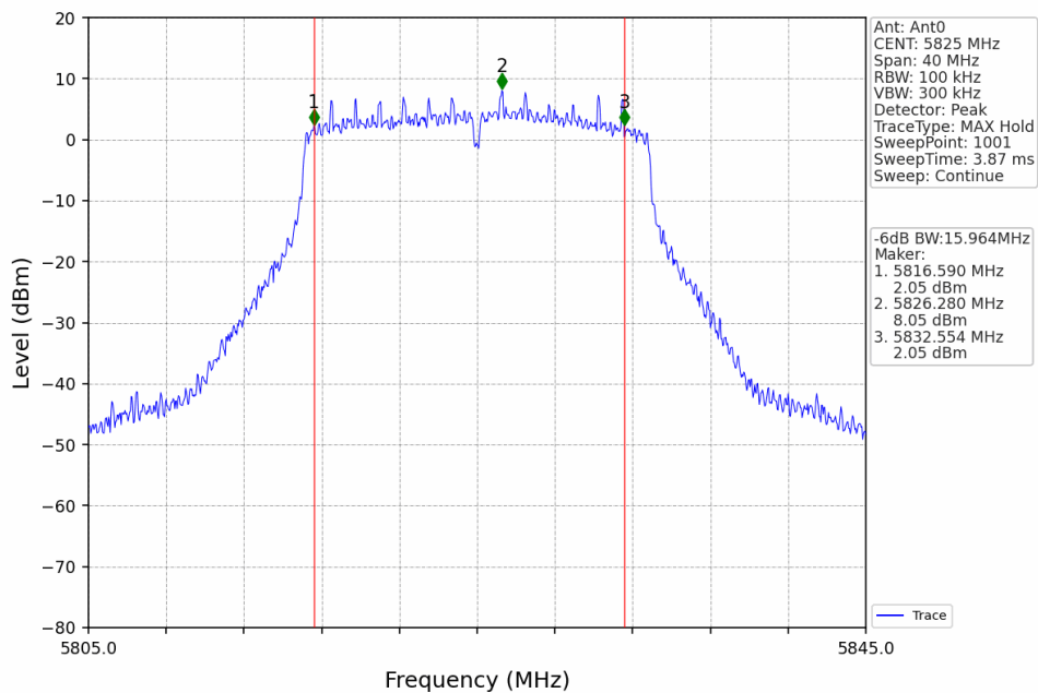
802.11n(HT20)_HCH_5825MHz_Ant0_NTNV
