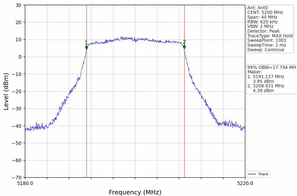
802.11ac(VHT20)_MCH_5200MHz_Ant0_NTNV
