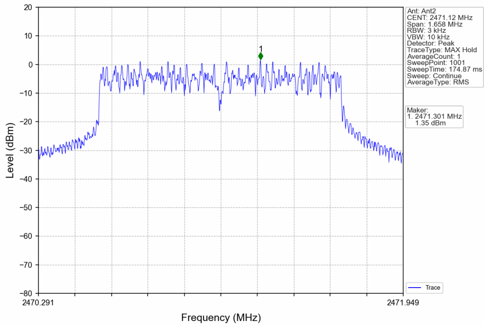
1.4M_HCH_2471.12MHz_Ant2_NTNV
