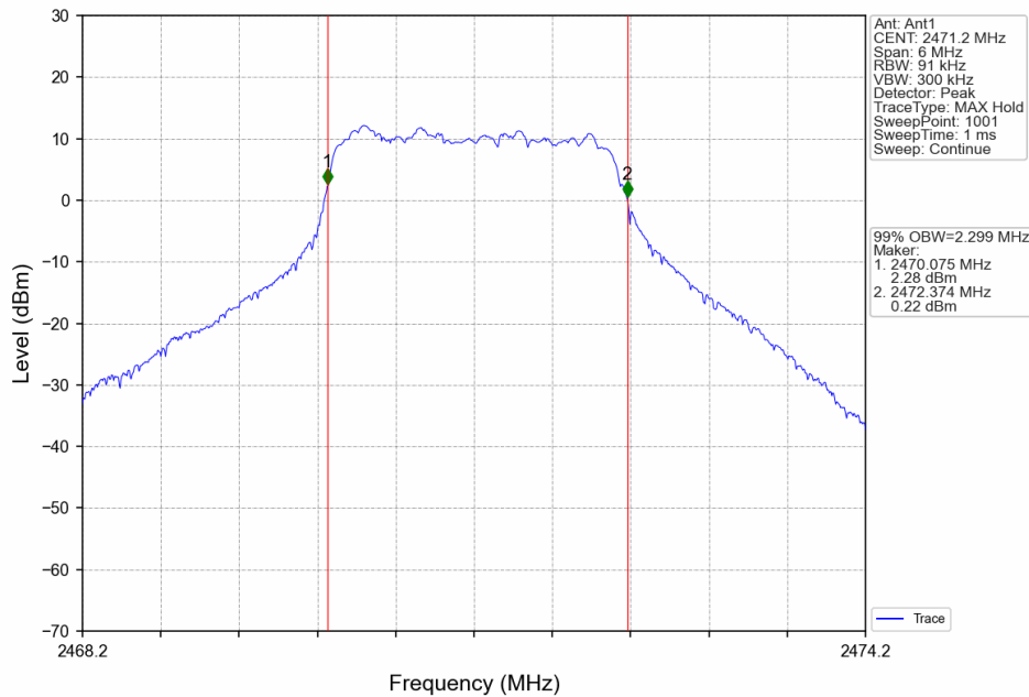
3M_HCH_2471.2MHz_Ant1_NTNV
