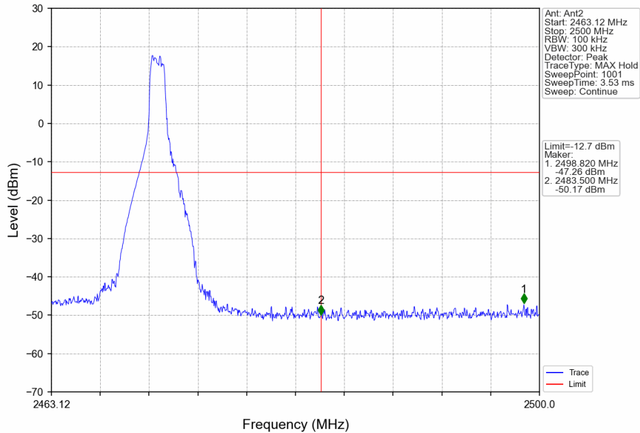
1.4M_HCH_2471.12MHz_Ant2_NTNV
