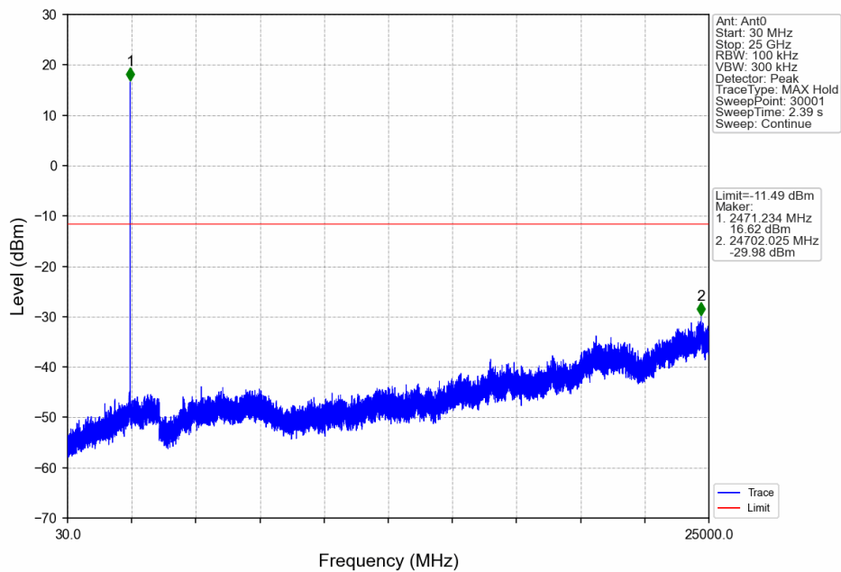
1.4M_HCH_2471.12MHz_Ant0_NTNV
