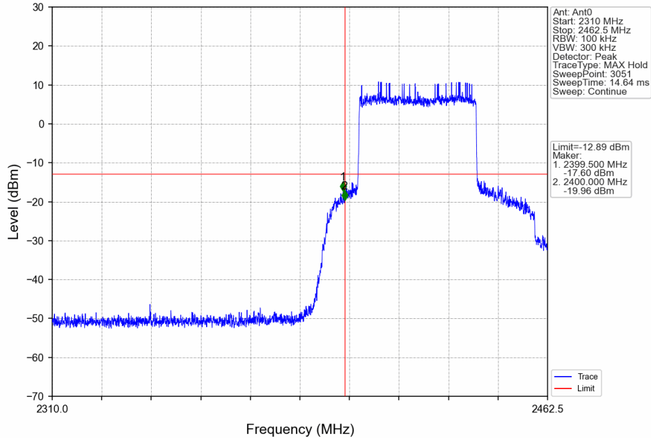
40M_LCH_2422.5MHz_Ant0_NTNV
