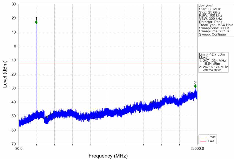
1.4M_HCH_2471.12MHz_Ant2_NTNV
