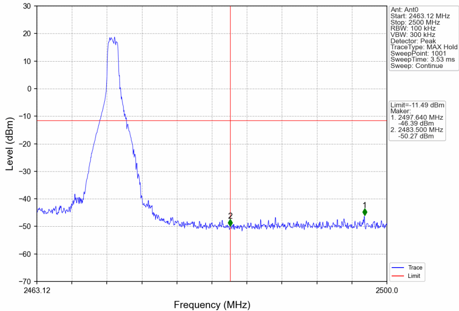
1.4M_HCH_2471.12MHz_Ant0_NTNV
