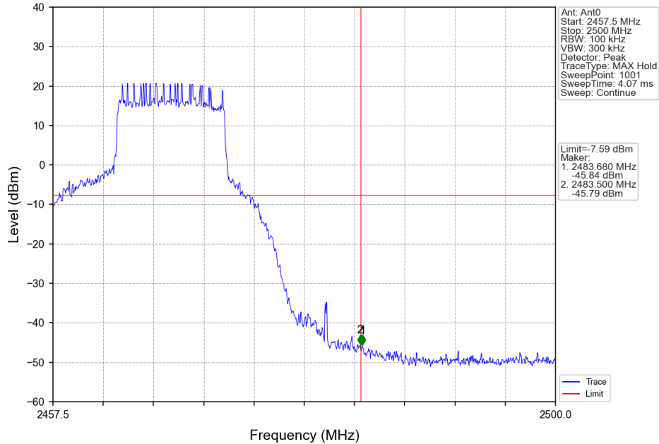
10M_HCH_2467.5MHz_Ant0_NTNV
