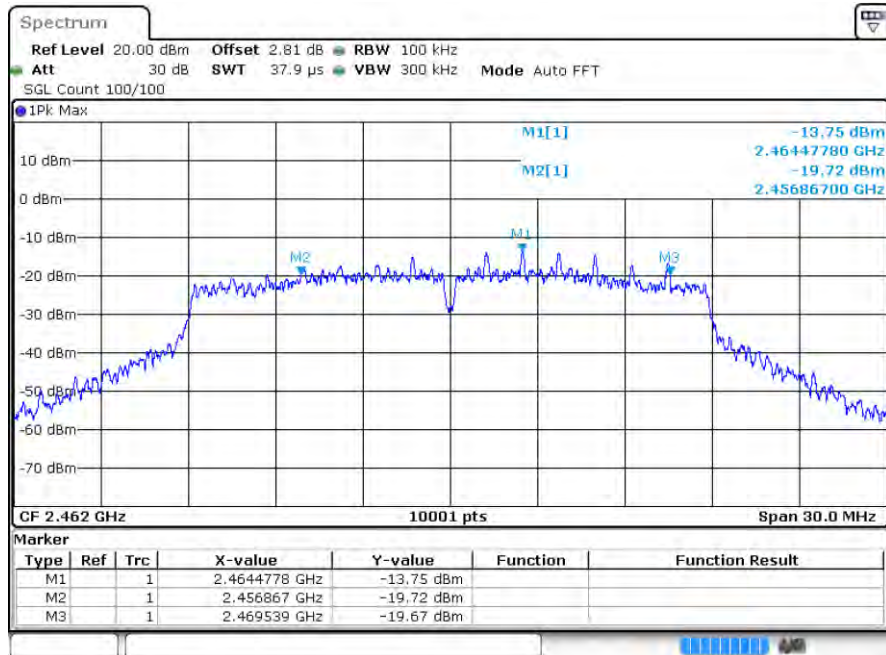
n20 2462MHz Ant1
