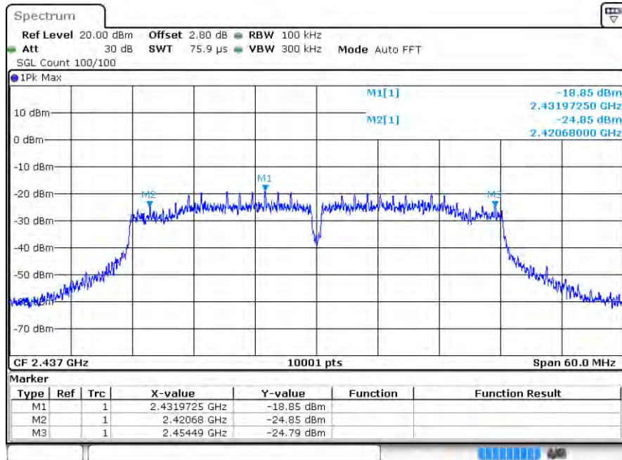
n40 2437MHz Ant1
