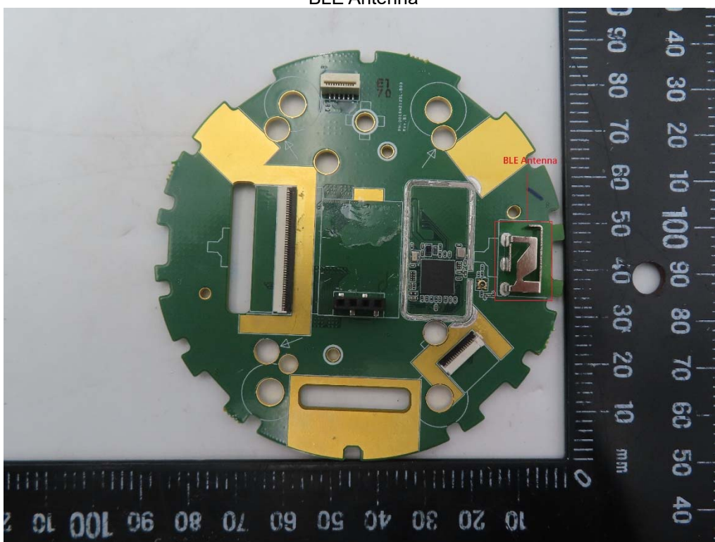
BLE Antenna
