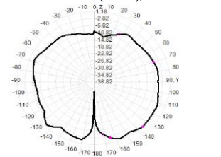
2490.0MHz Total(E2-YZ), Max= -3.03dBi
