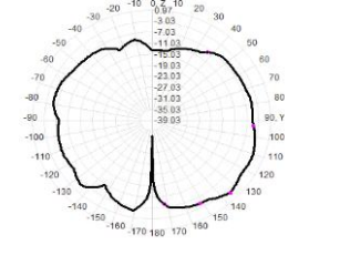
2430.0MHz Total(E2-YZ), Max= -1.96dBi
