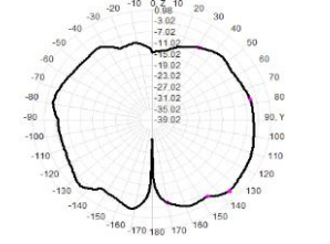
2460.0MHz Total(E2-YZ), Max= -2.34dBi
