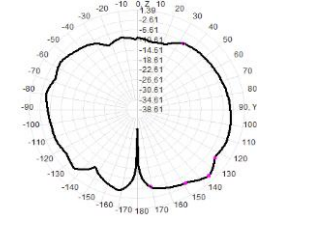
2410.0MHz Total(E2-YZ), Max= -1.00dBi
