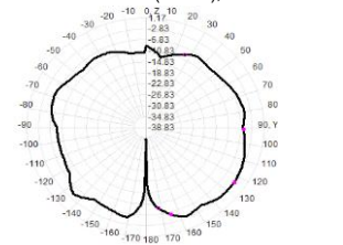
2500.0MHz Total(E2-YZ), Max= -2.57dBi
