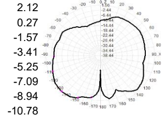
2420.0MHz Total(E1-XZ), Max= 1.41dBi
