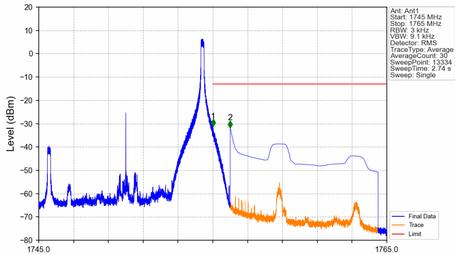
Band4_10MHz_QPSK_HCH_1750MHz_RB_1_49_NTNV
