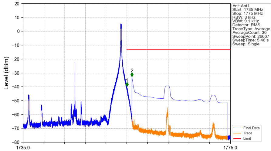
Band4_20MHz_QPSK_HCH_1745MHz_RB_1_99_NTNV
