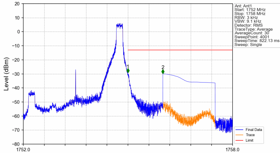
Band4_3MHz_QPSK_HCH_1753.5MHz_RB_1_14_NTNV
