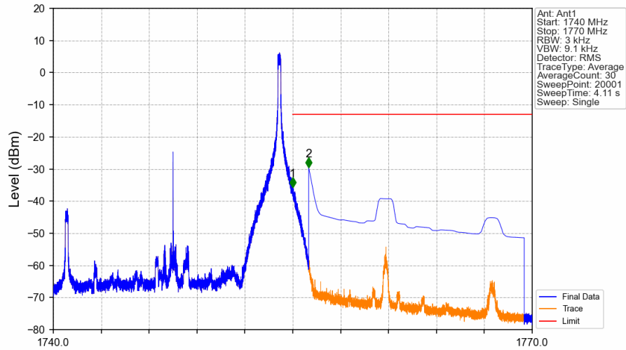
Band4_15MHz_QPSK_HCH_1747.5MHz_RB_1_74_NTNV
