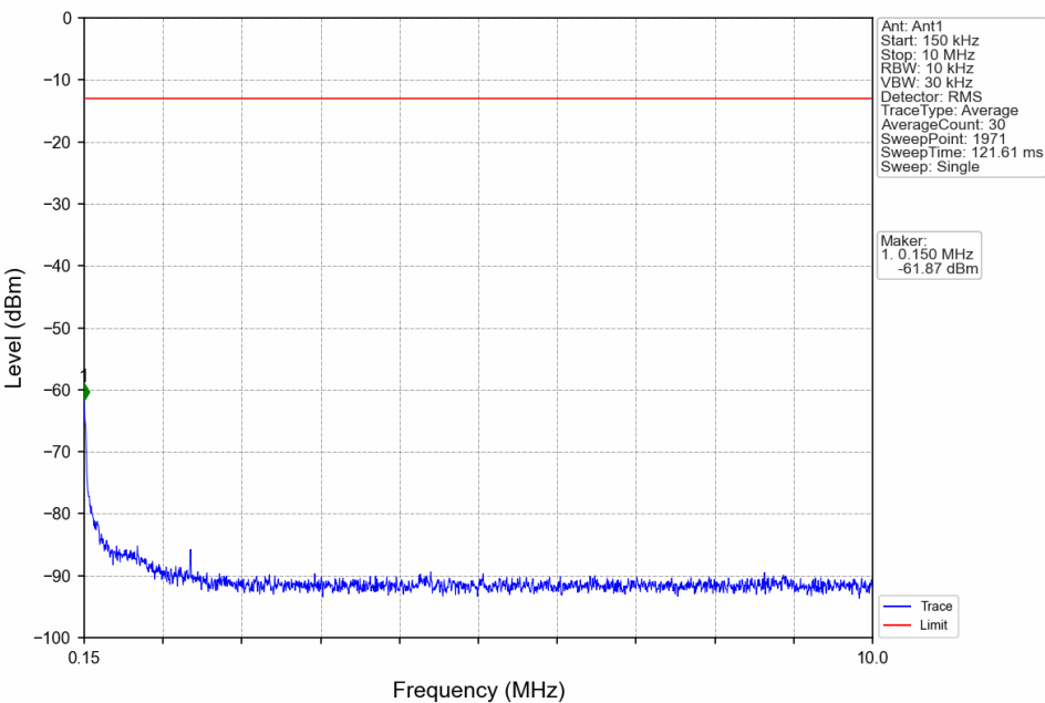
Band4_10MHz_QPSK_HCH_1750MHz_RB_1_49_NTNV
