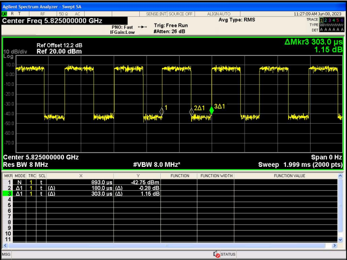
IEEE 802.11a_20MHz_Channel 165
