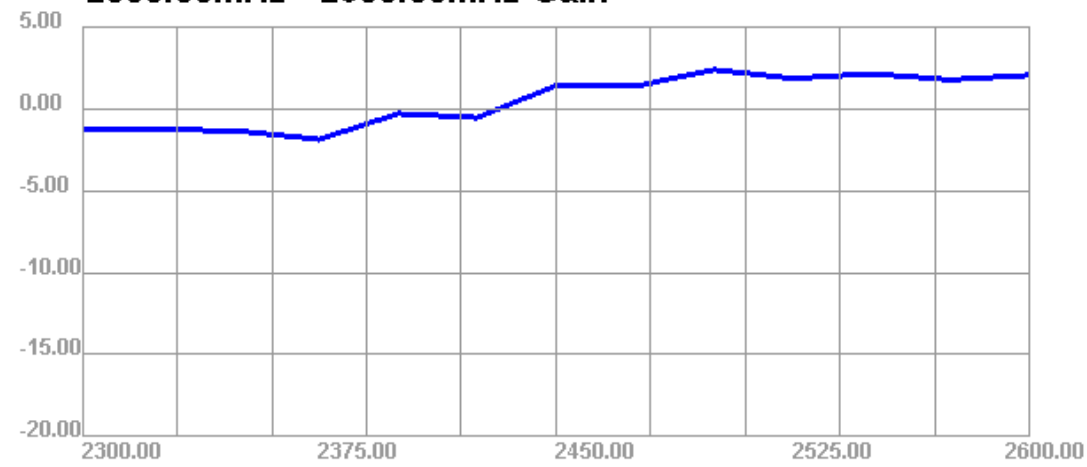
2300.00MHz - 2600.00MHz Gain
