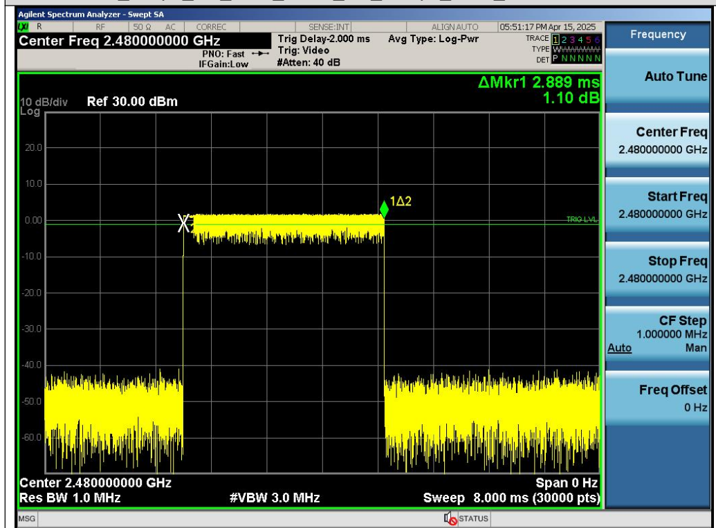
Test_Graph_BR_HOP_ANT1_NA_2Mbps_2480_Time per Burst
