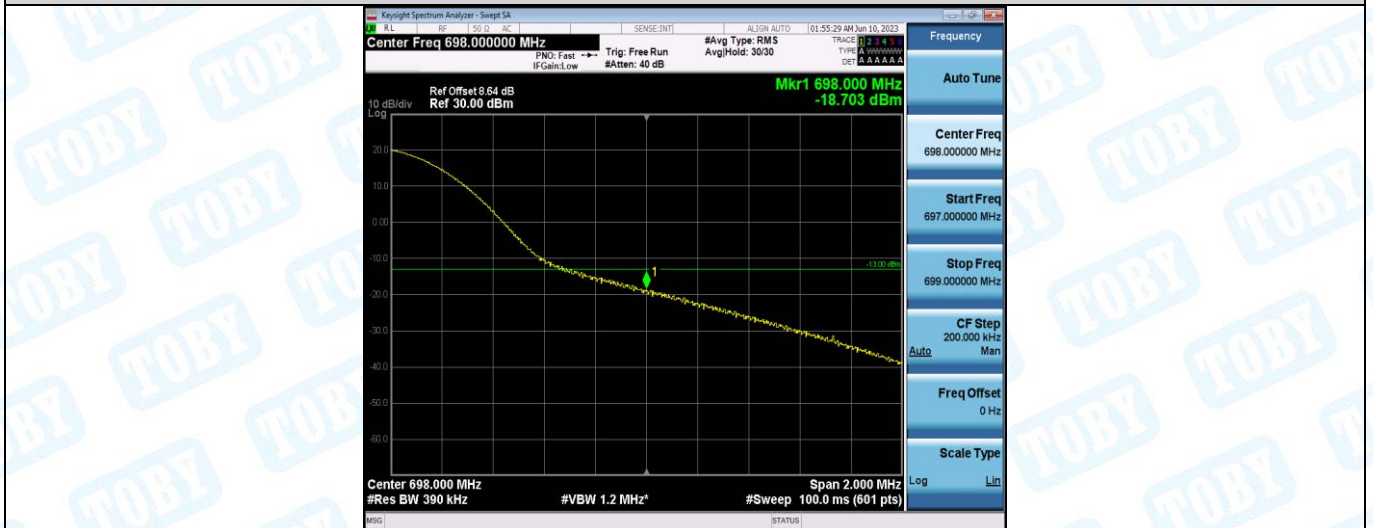
Band71-20MHz-QPSK-133372-100RB#0
