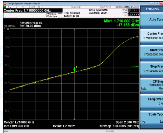
Band66-20MHz-QPSK-132072-1RB#99
