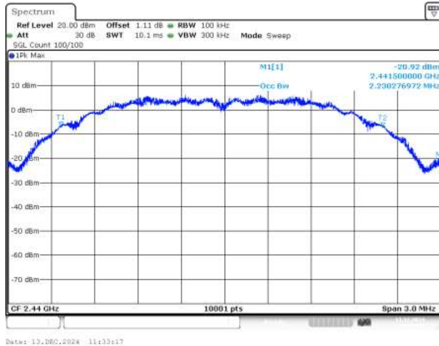
OBW 2440MHz Ant1
