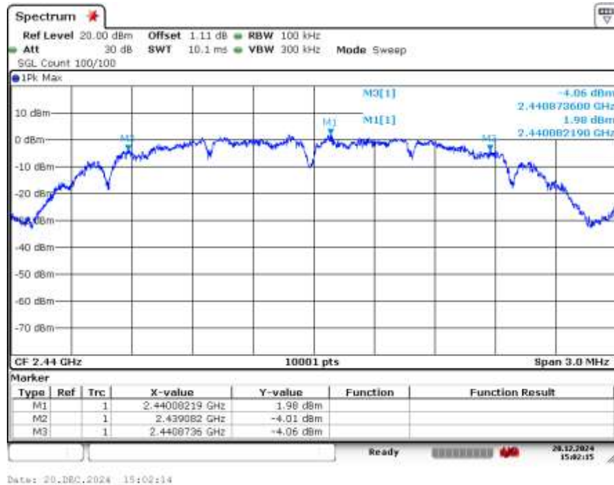
-6dB Bandwidth 2440MHz Ant1
