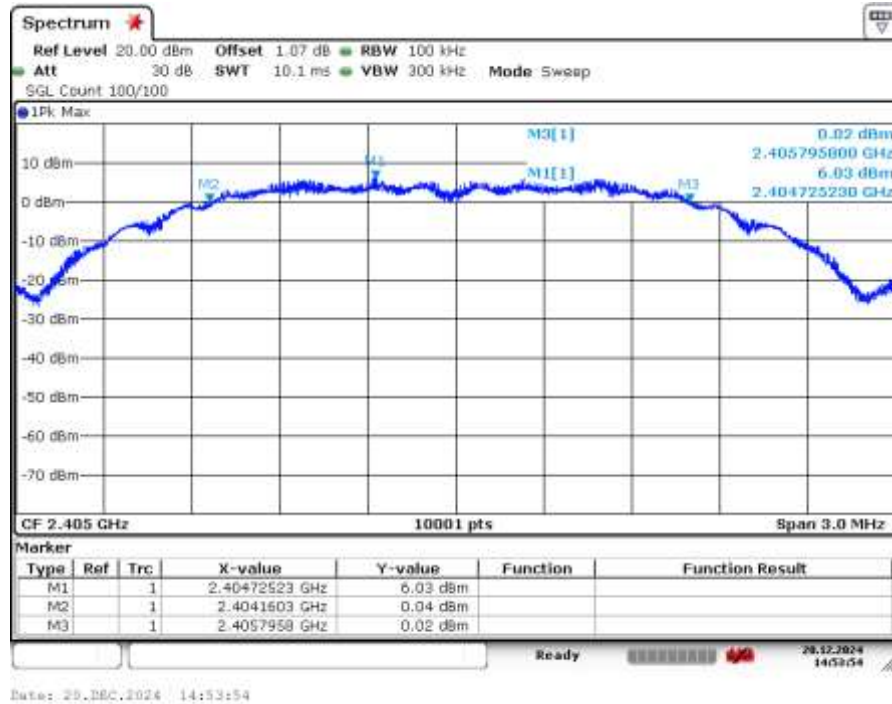
-6dB Bandwidth 2405MHz Ant1
