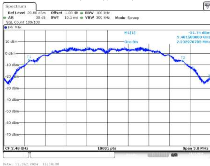
OBW 2480MHz Ant1
