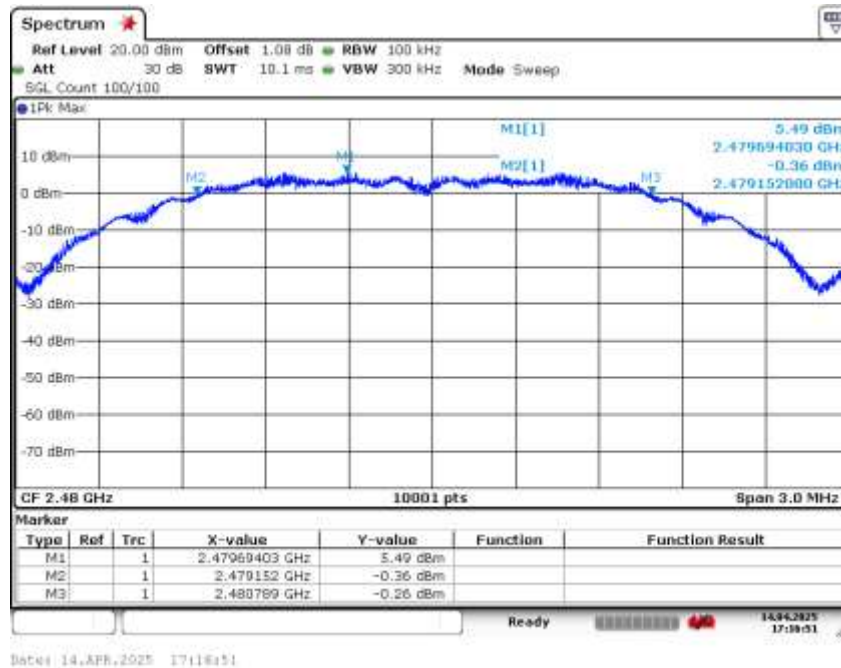
-6dB Bandwidth 2480MHz Ant1
