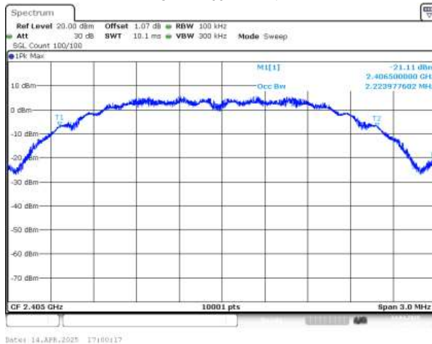
OBW 2405MHz Ant1
