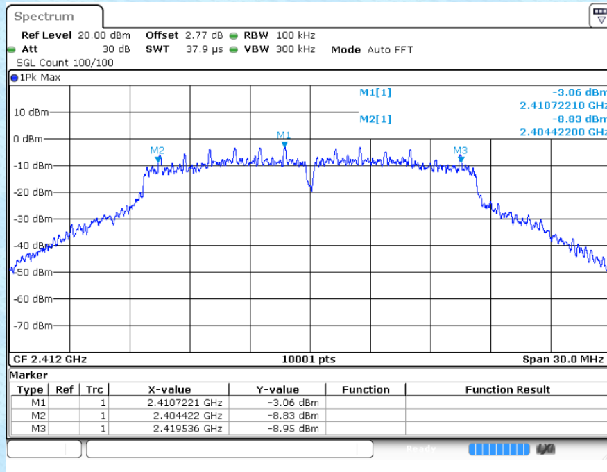
g 2412MHz Ant1
