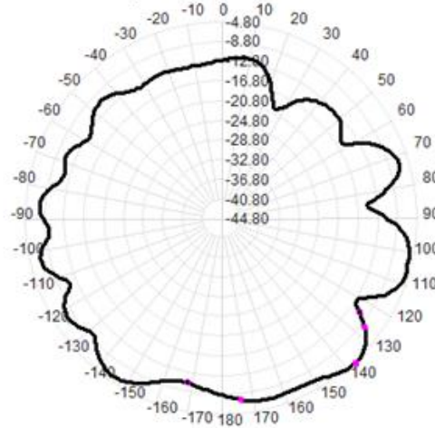
2472.0MHz Total(E2-YZ), Max= -4.80dBi
