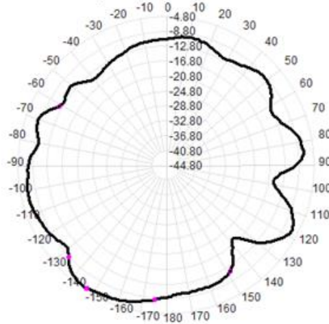
2472.0MHz Total(E1-XZ), Max= -5.63dBi
