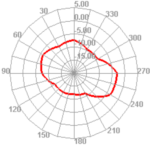
2400.000MHz H
