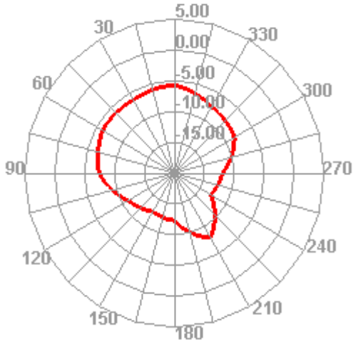
2400.000MHz E1
