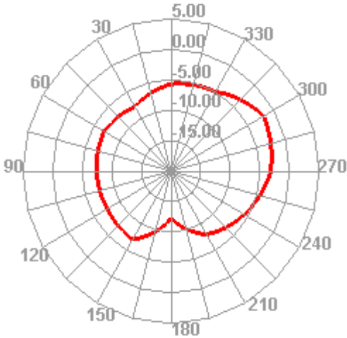
2400.000MHz E2
