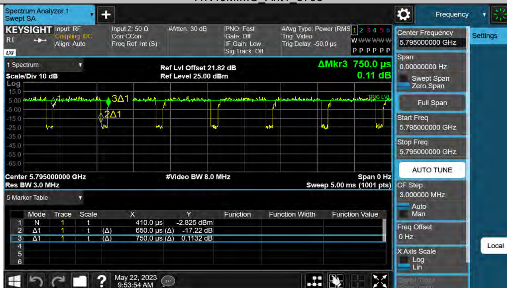
11N40MIMO Ant1 5795
