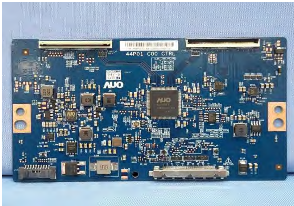
EUT Photo (72)
