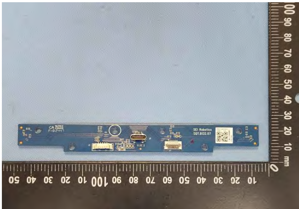
EUT Photo (82)
