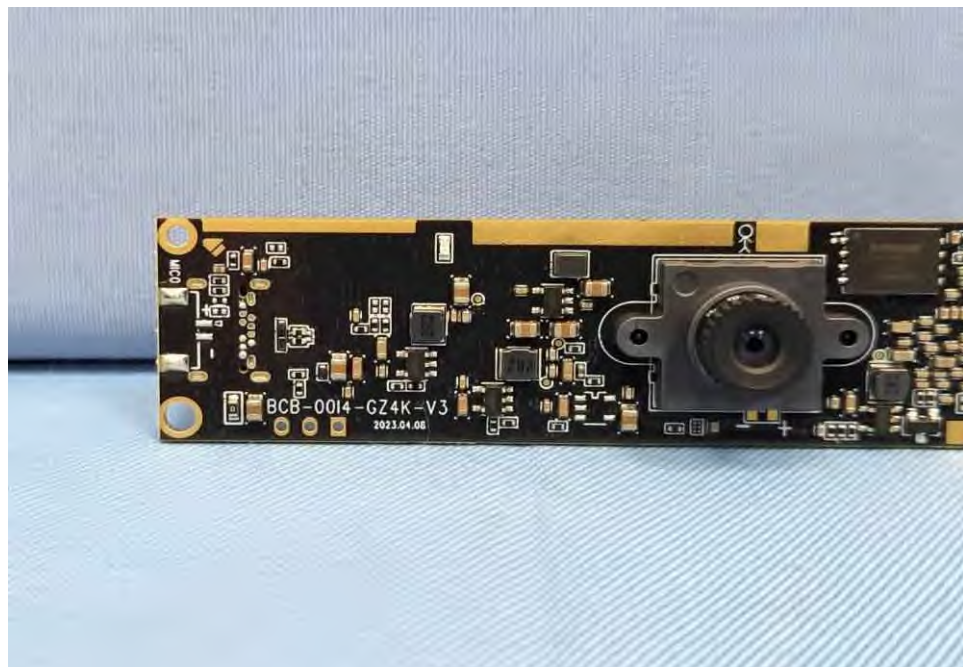
EUT Photo (112)
