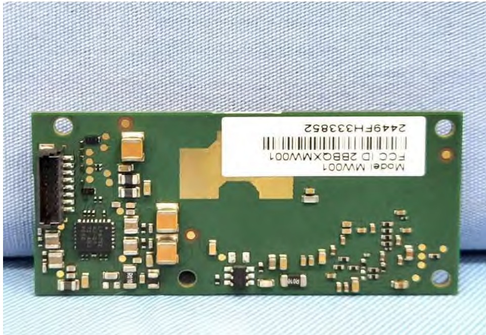
EUT Photo (104)
