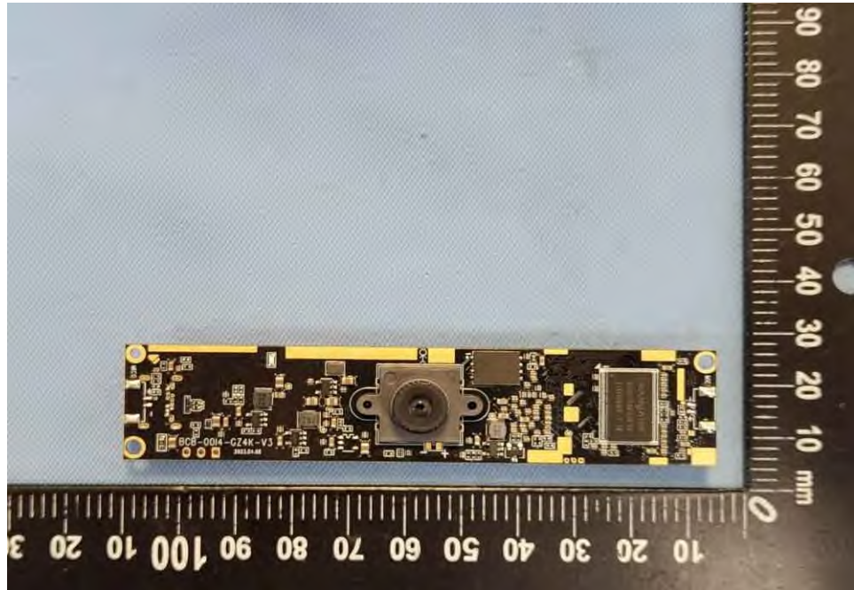
EUT Photo (112)
