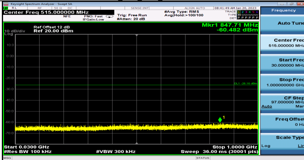
11G_Ant1_2462_30-1000
