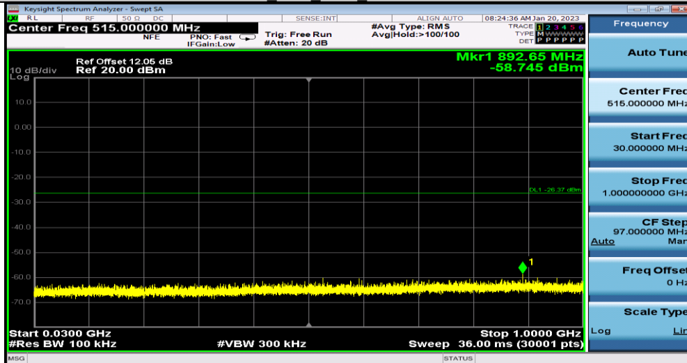
11G_Ant1_2412_30-1000
