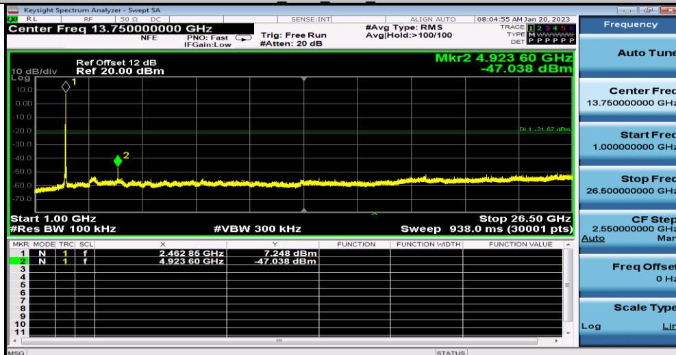
11B_Ant1_2462_1000-26500
