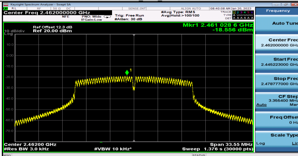
11G_Ant1_2462
