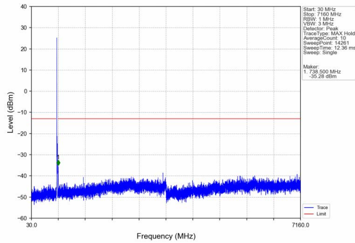
Band12_10MHz_QPSK_MCH_707.5MHz_RB_1_0_NTNV
