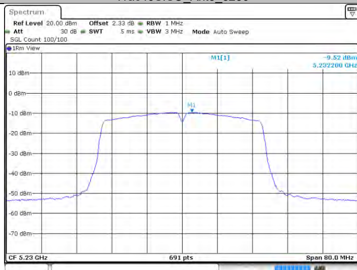
11ac40SISO_Ant3_5230
