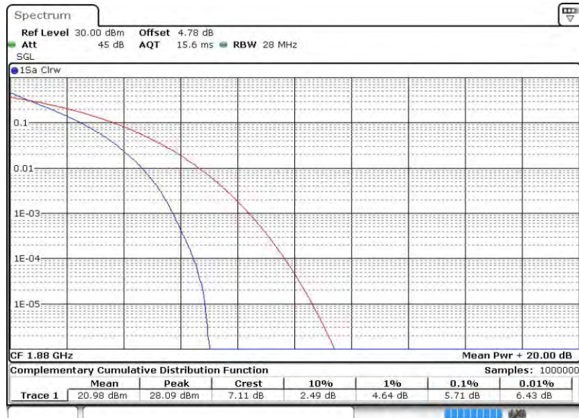
Band2-20MHz-QPSK-18900-100RB#0
