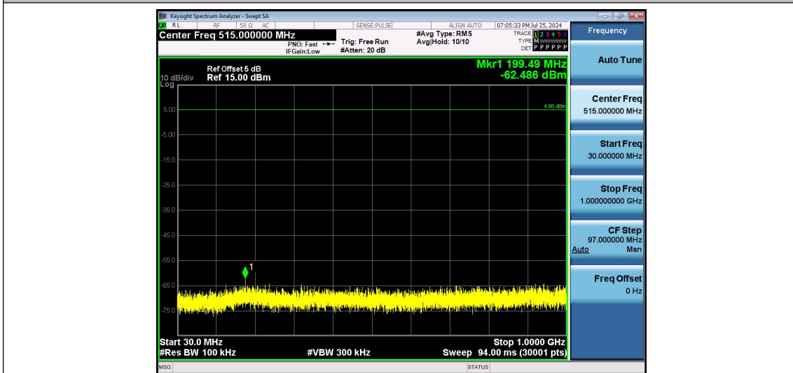
2.4G-Ant1-2402.4-30~1000-PASS
