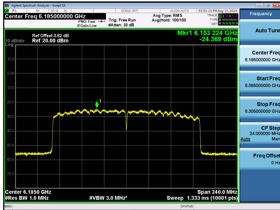
PSD NVNT ax160 6185MHz Ant2
