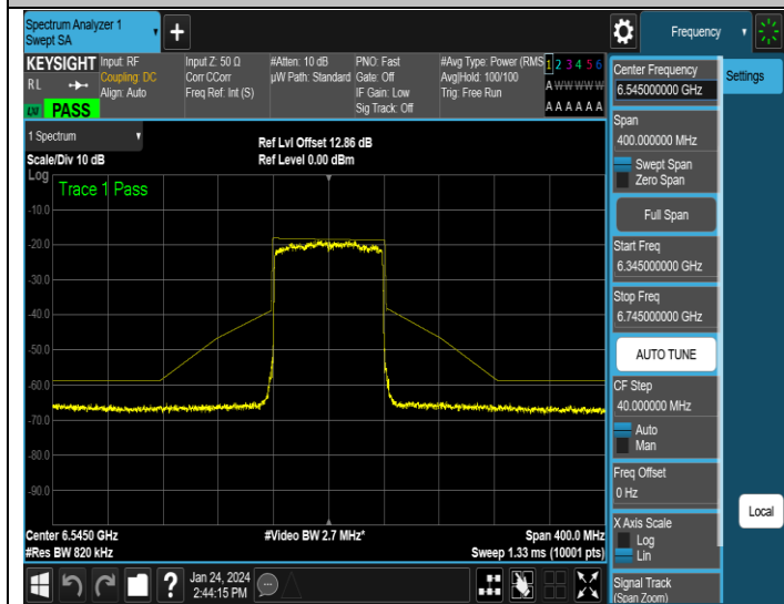
NTVN-11AX80MIMO-Ant1-6545-PASS
