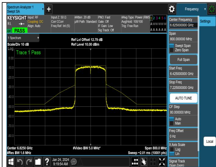
NTNV-11AX160SISO-Ant1-6825-PASS
