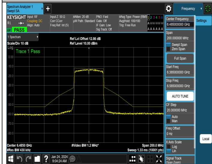
NTNV-11AX40ISO-Ant1-6485-PASS
