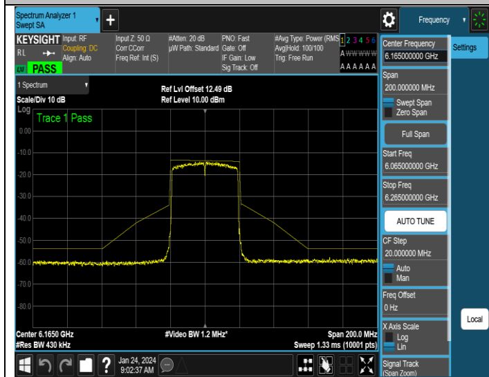
NTNV-11AX40ISO-Ant1-6165-PASS
