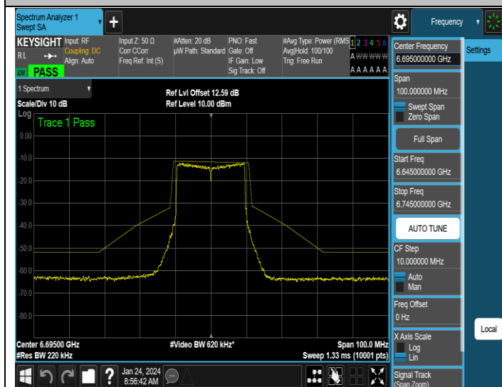
NTNV-11AX20SISO-Ant1-6695-PASS
