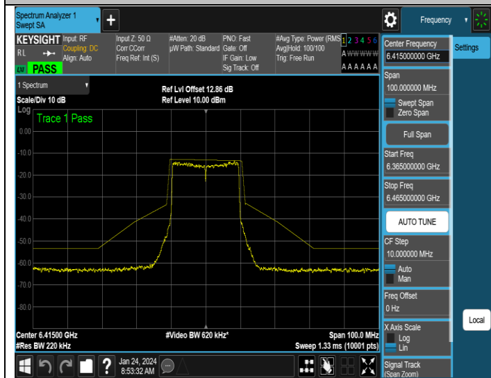
NTNV-11AX20SISO-Ant1-6415-PASS
