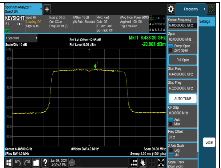
11AX40MIMO-Ant4-6485-PASS
