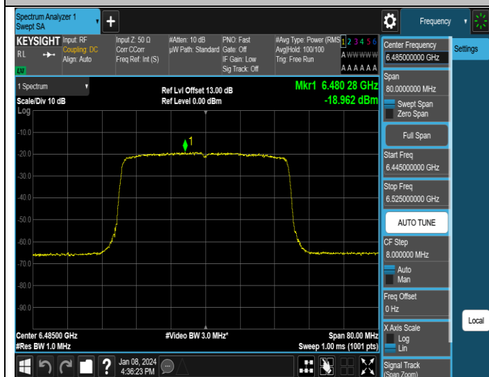
11AX40MIMO-Ant1-6485-PASS
