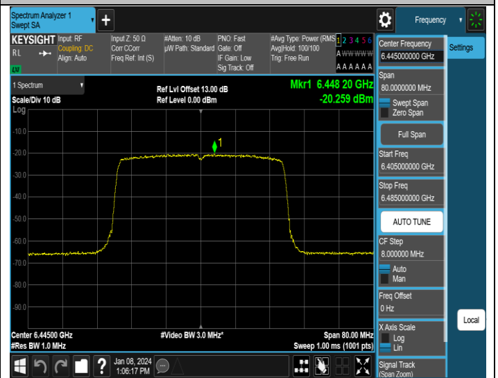
11AX40MIMO-Ant4-6445-PASS
