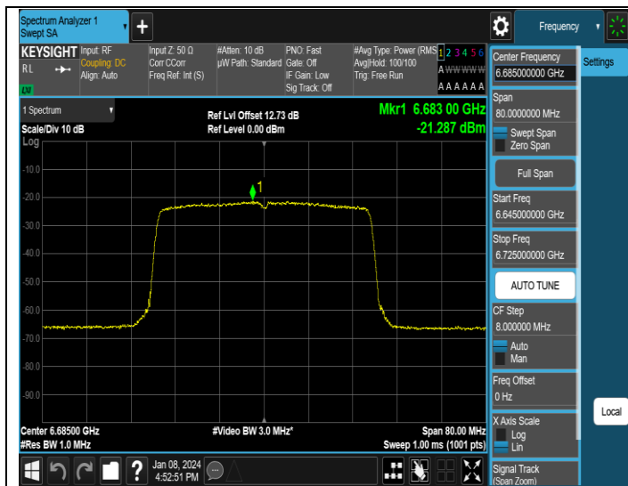
11AX40MIMO-Ant3-6685-PASS
