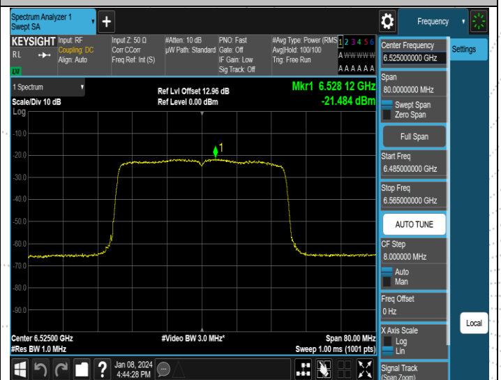
11AX40MIMO-Ant4-6525-PASS
