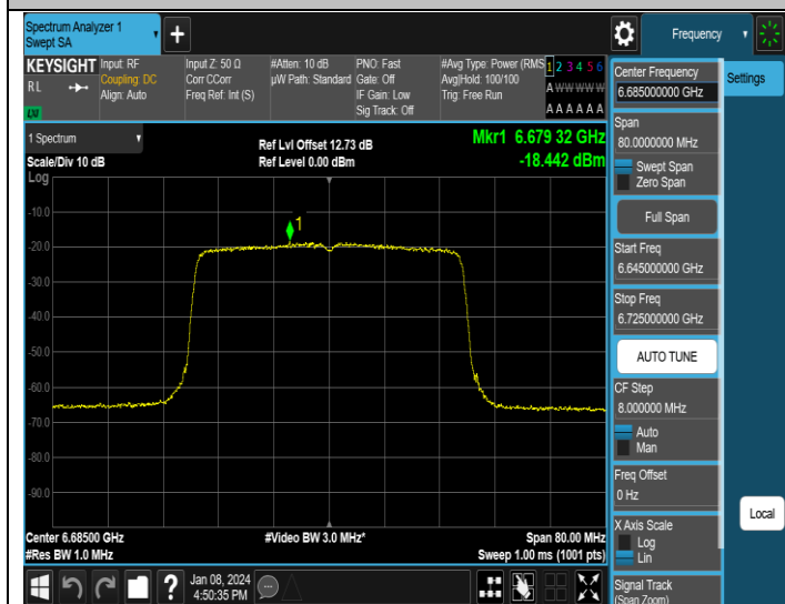
11AX40MIMO-Ant1-6685-PASS
