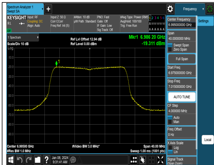
11AX20MIMO-Ant3-6995-PASS
