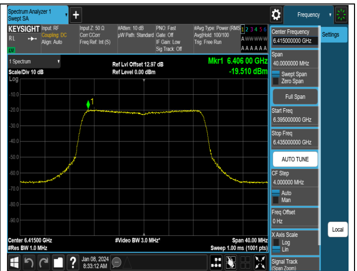
11AX20MIMO-Ant4-6415-PASS
