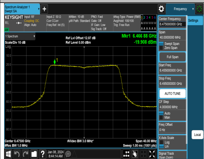
11AX20MIMO-Ant4-6475-PASS
