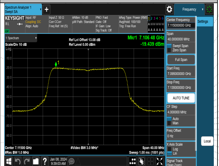
11AX20MIMO-Ant4-7115-PASS
