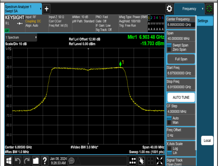
11AX20MIMO-Ant4-6895-PASS
