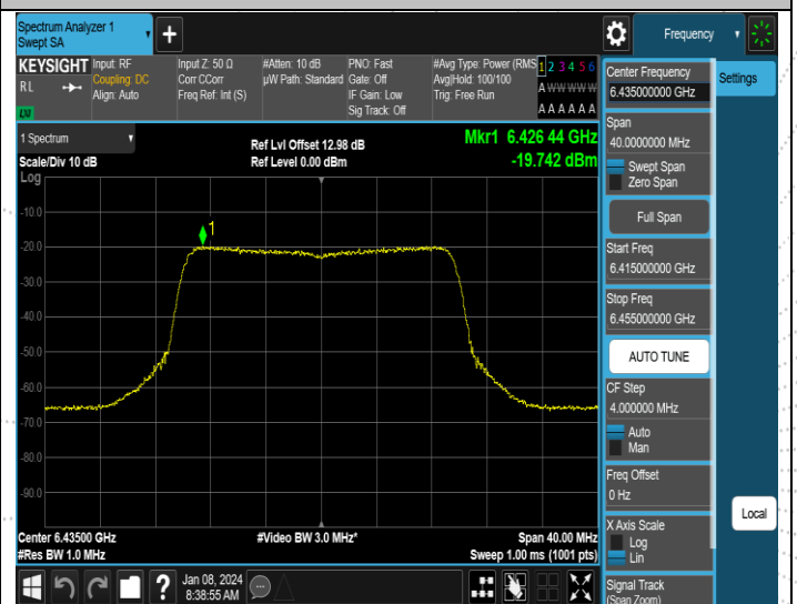
11AX20MIMO-Ant4-6435-PASS
