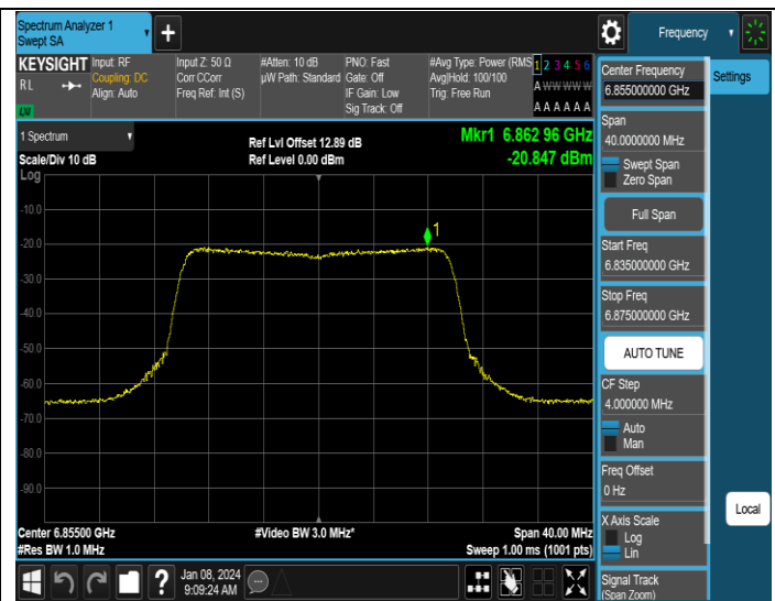
11AX20MIMO-Ant4-6855-PASS
