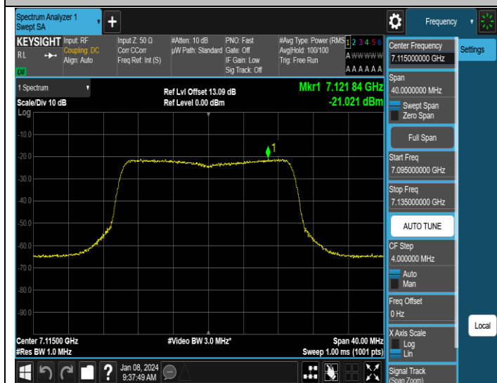
11AX20MIMO-Ant3-7115-PASS
