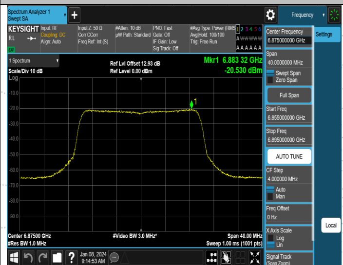
11AX20MIMO-Ant4-6875-PASS
