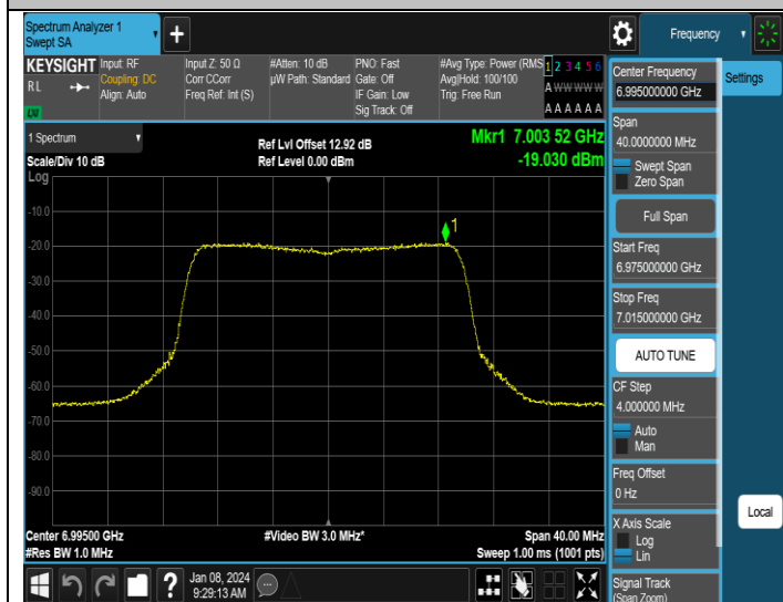
11AX20MIMO-Ant1-6995-PASS
