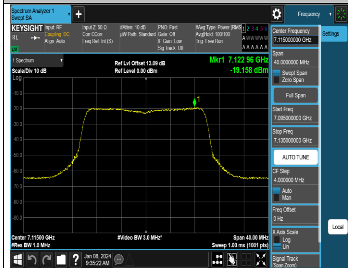
11AX20MIMO-Ant1-7115-PASS
