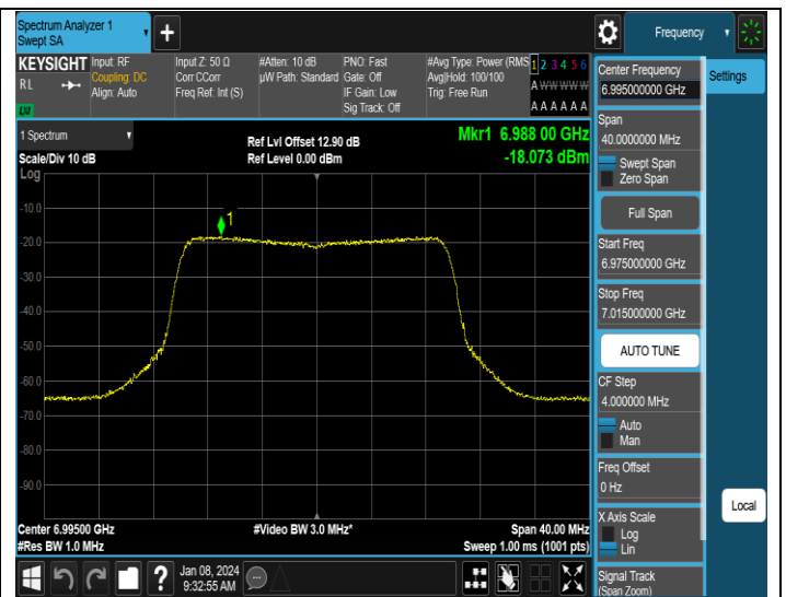
11AX20MIMO-Ant4-6995-PASS
