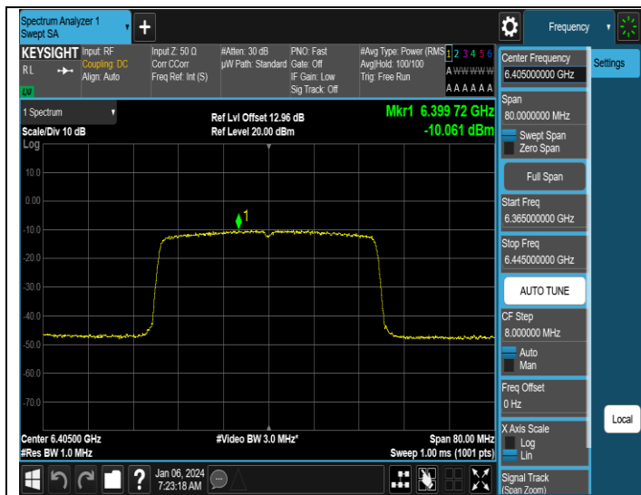
11AX40SISO-Ant1-6405-PASS
