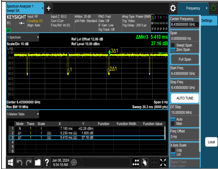
NTNV-11AX20MIMO-Ant1-6435
