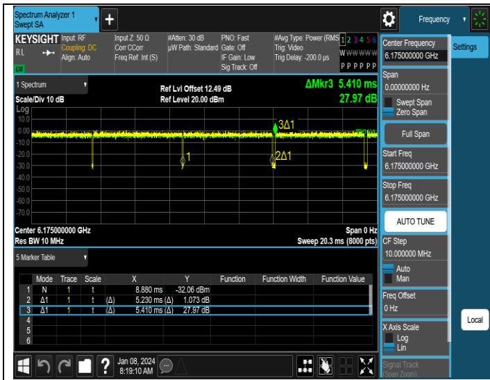
NTNV-11AX20MIMO-Ant1-6175
