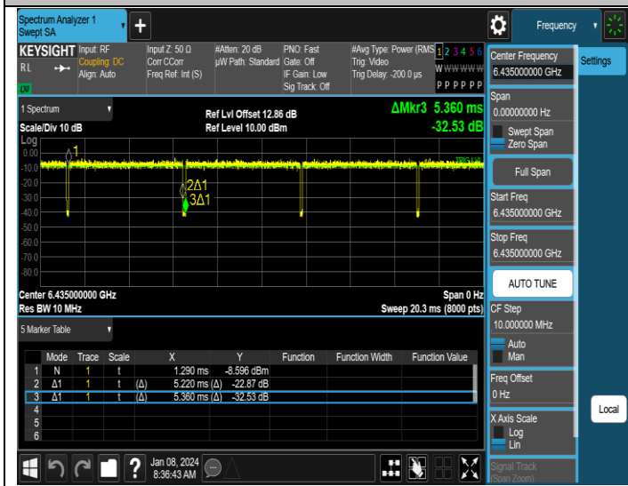
NTNV-11AX20MIMO-Ant3-6435
