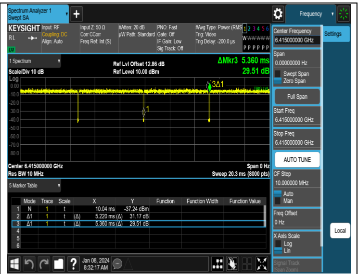
NTNV-11AX20MIMO-Ant4-6415
