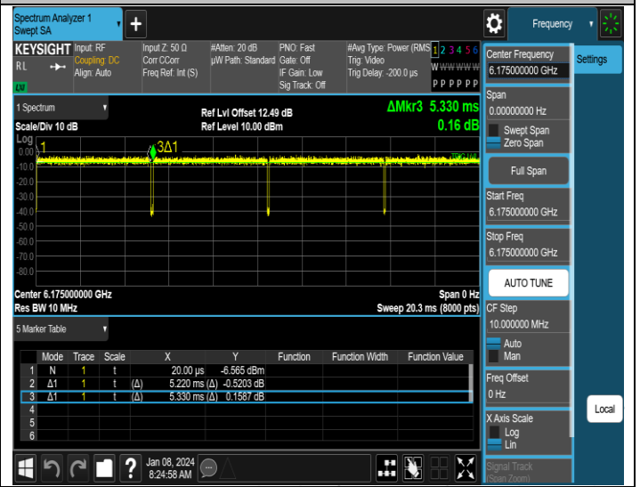
NTNV-11AX20MIMO-Ant4-6175
