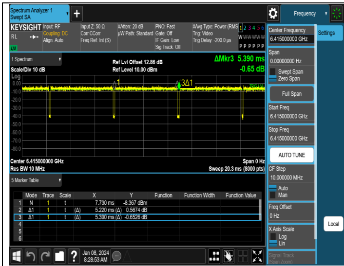
NTNV-11AX20MIMO-Ant3-6415
