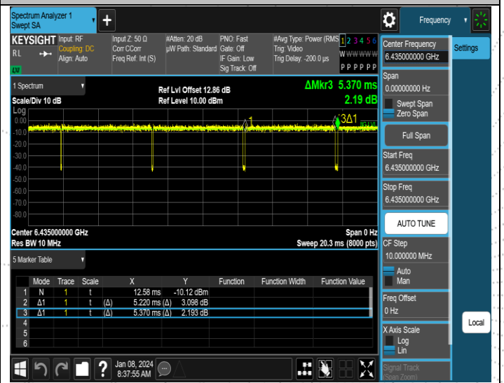
NTNV-11AX20MIMO-Ant4-6435
