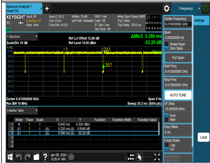
NTNV-11AX20MIMO-Ant1-6415
