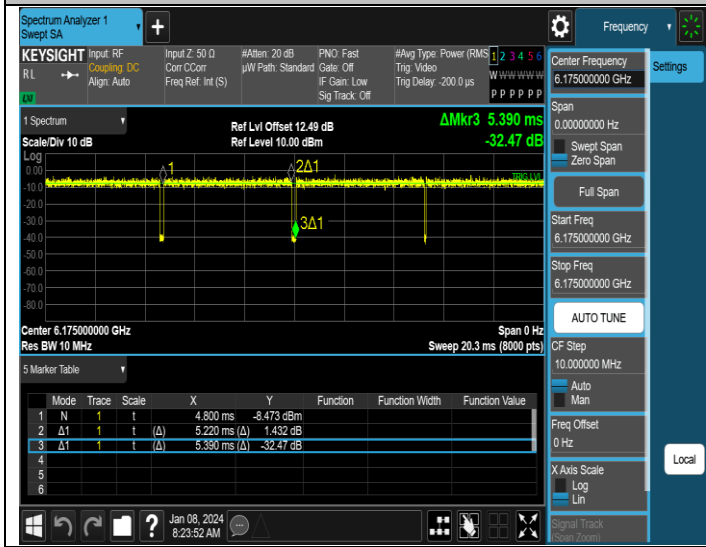
NTNV-11AX20MIMO-Ant3-6175
