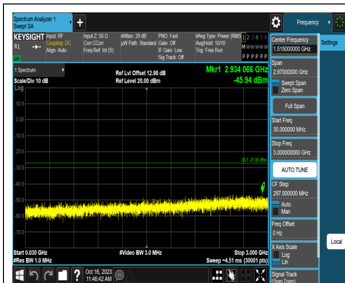
11AX20MIMO-Ant3-7115-30~3000-PASS
