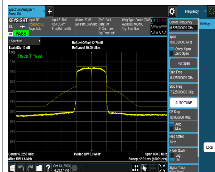
NTNV-11AX160SISO-Ant1-6825-PASS
