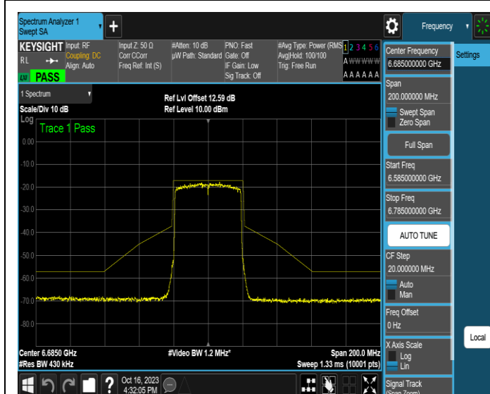
NTNV-11AX40MIMO-Ant1-6685-PASS
