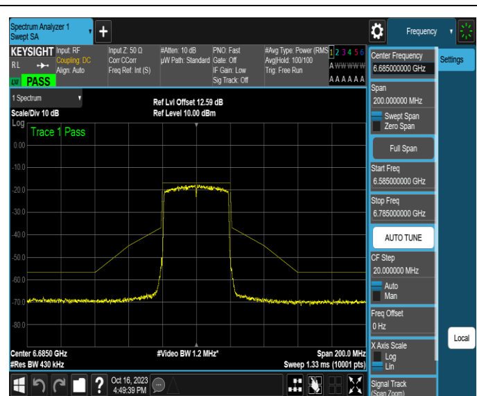
NTNV-11AX40MIMO-Ant4-6685-PASS
