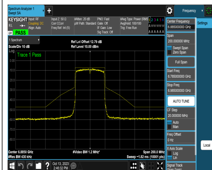
NTNV-11AX40SISO-Ant1-6885-PASS
