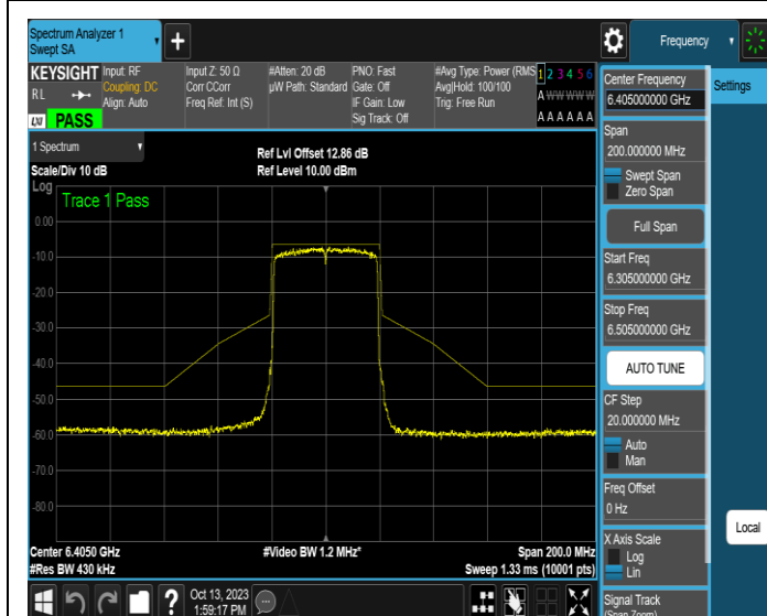
NTNV-11AX40SISO-Ant1-6405-PASS
