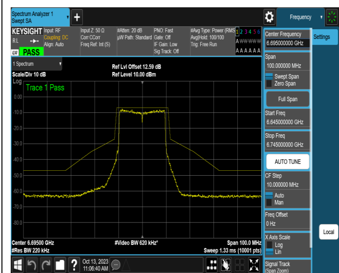
NTNV-11AX20SISO-Ant1-6695-PASS
