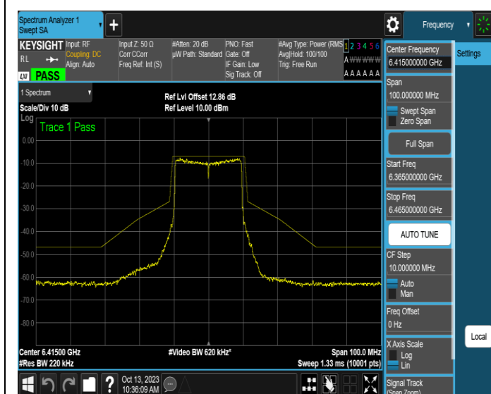
NTNV-11AX20SISO-Ant1-6415-PASS
