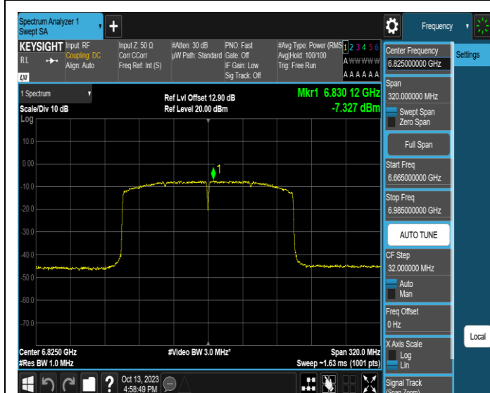
11AX160SISO-Ant1-6825-PASS
