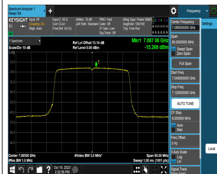
11AX40MIMO-Ant3-7085-PASS
