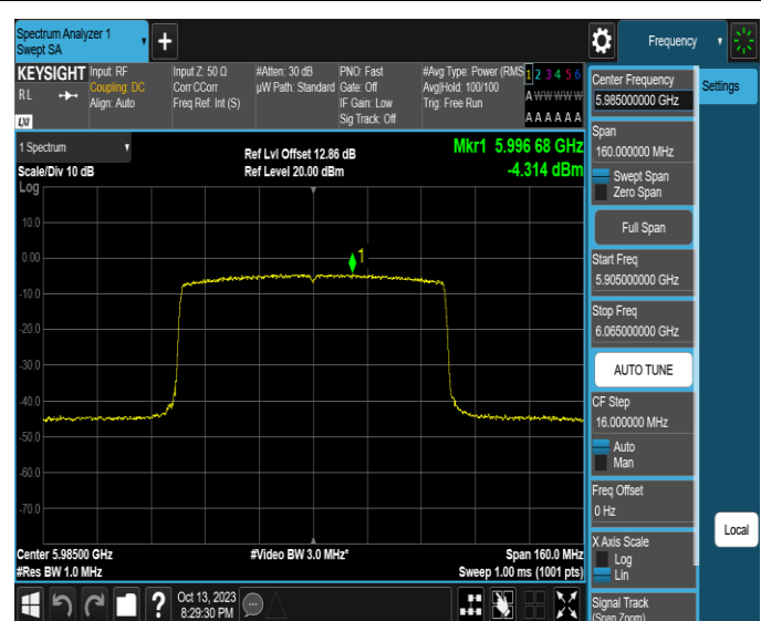
11AX80SISO-Ant2-5985-PASS
