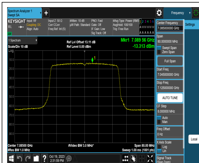
11AX40MIMO-Ant1-7085-PASS
