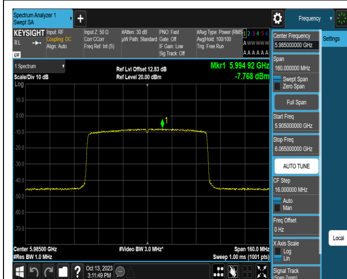
11AX80SISO-Ant1-5985-PASS
